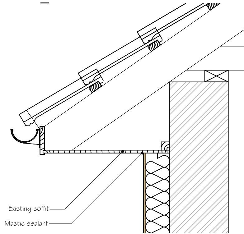
DO5_A - EAVES
