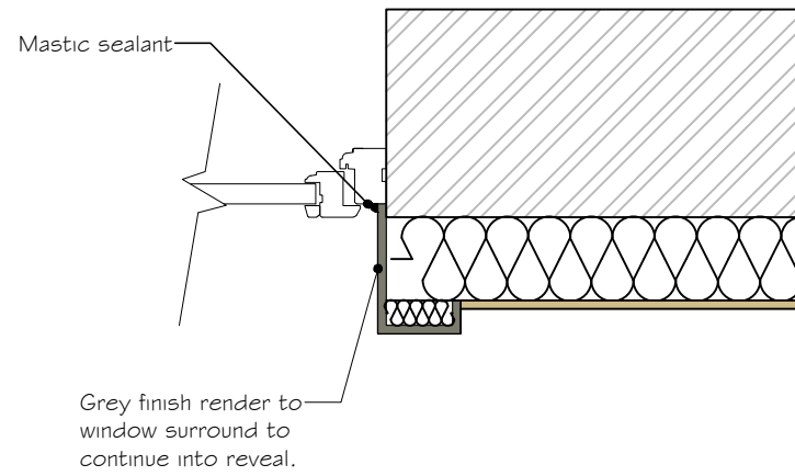
DOI_D - WINDOW JAMB
