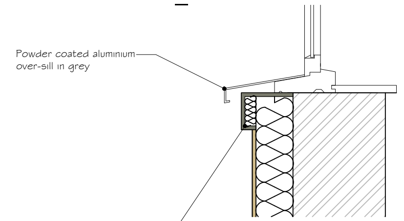
DOI_F - WINDOW SILL
