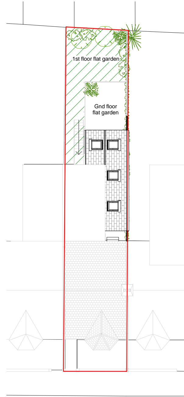
2 Site Plan 1 : 200
