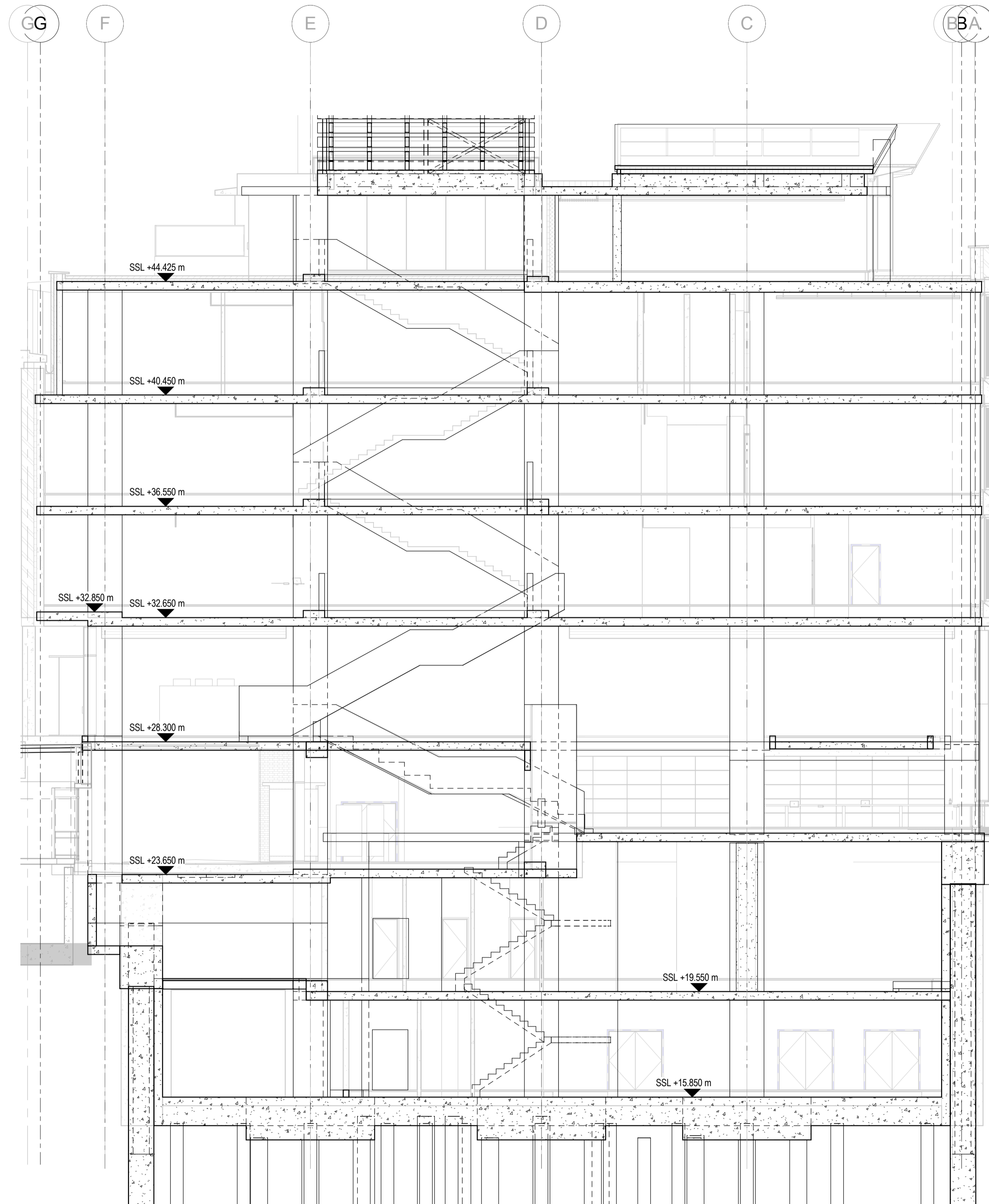
B SECTION B-B 1 : 100
