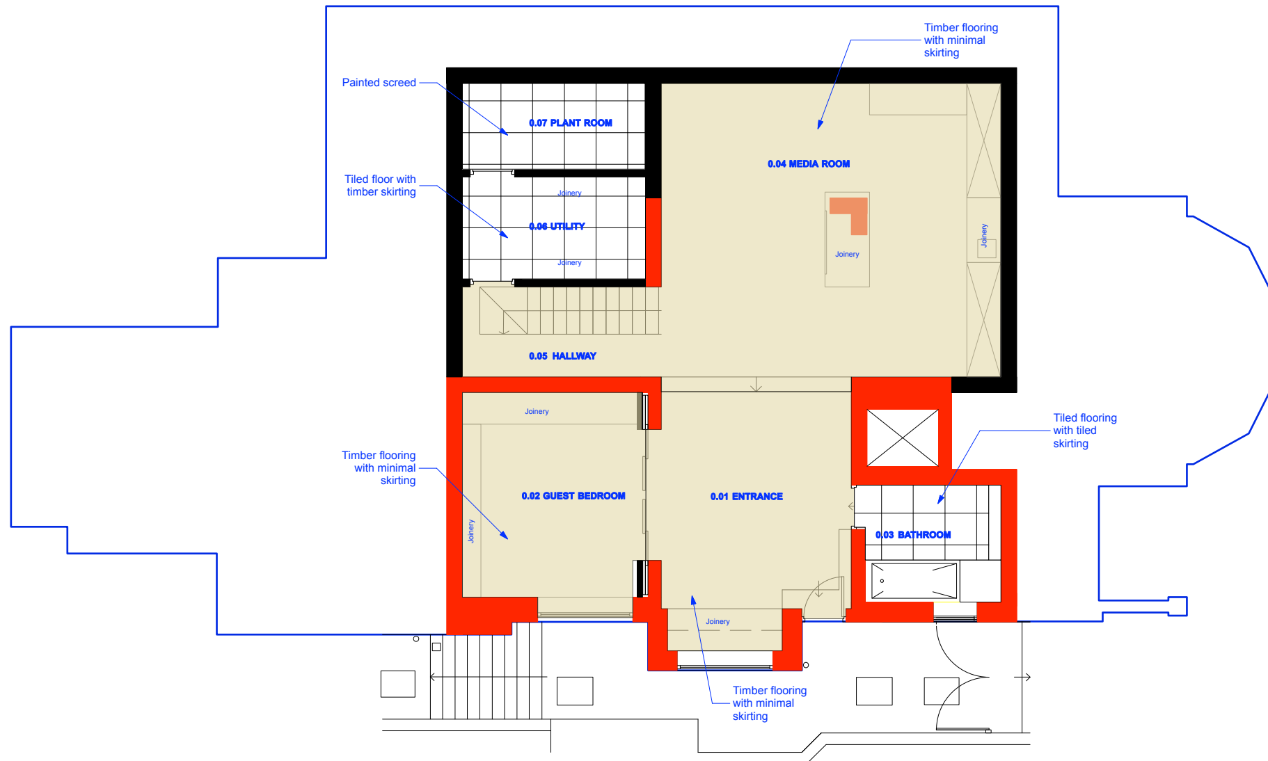
1 FLOOR FINISHES PLAN - GIA:93m2 Scale: 1:50
