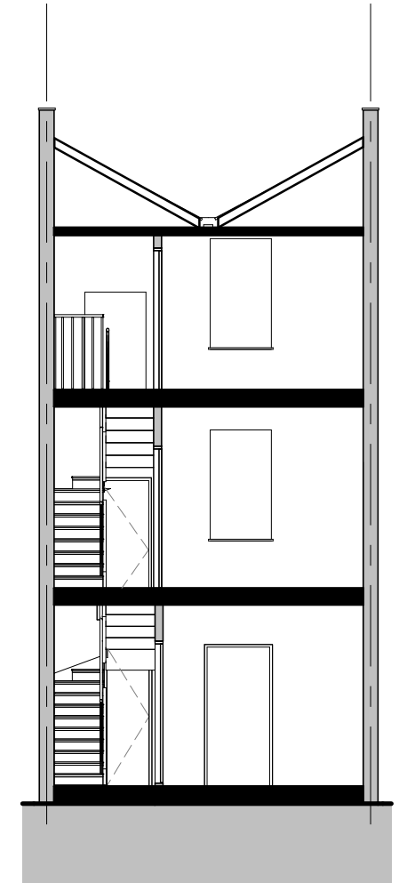
3 Section 2-2 1 : 100
