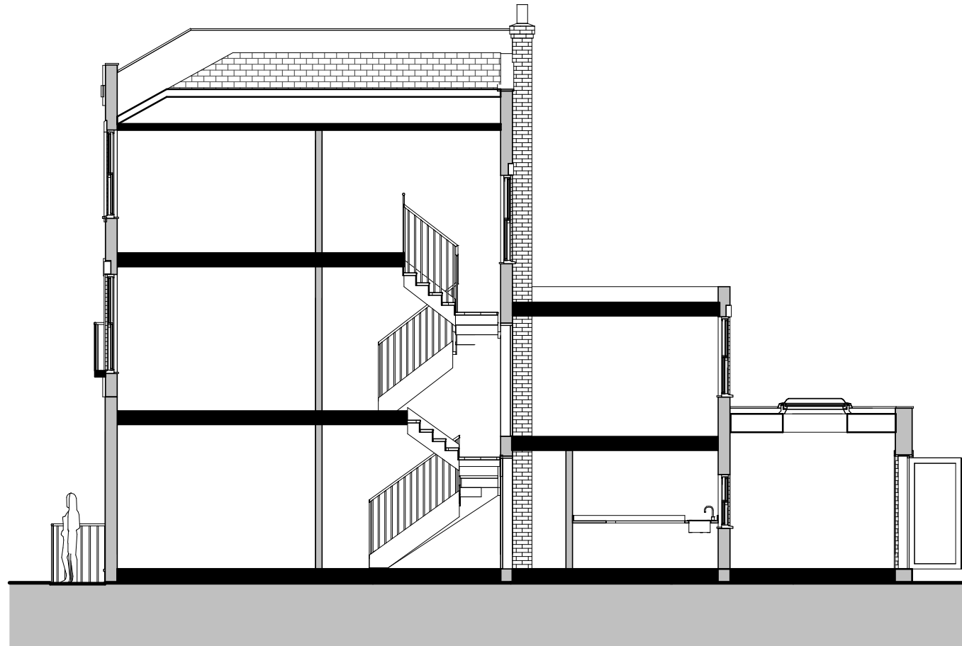
4 Section 1-1 1 : 100
