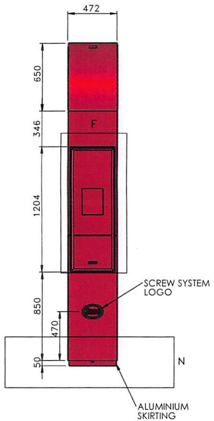
SECTION R-R SCALE 1 : 25
