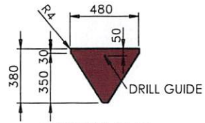
SECTION R-R SCALE 1 : 25
