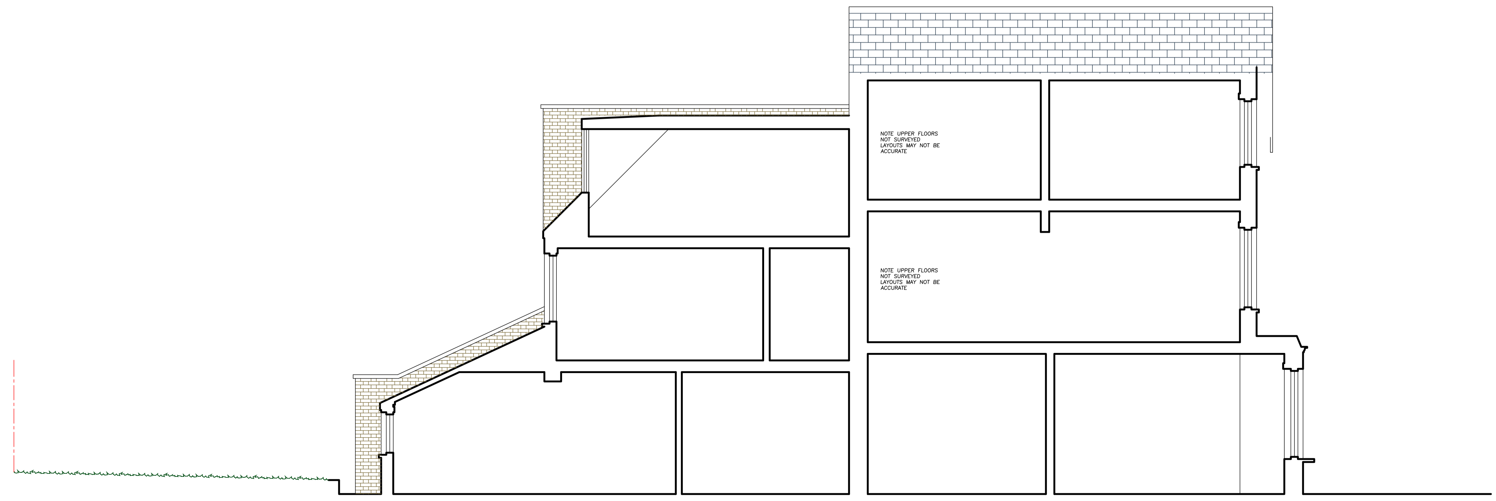
SECTION A-A
