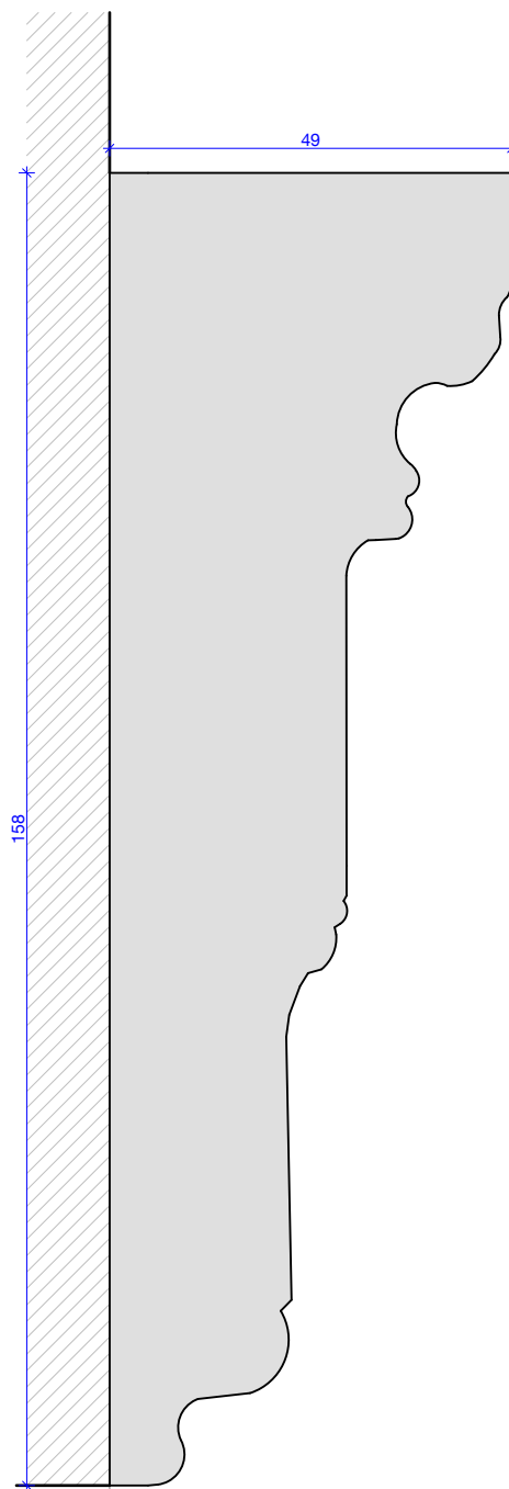
1:1 Door Architrave Profile
