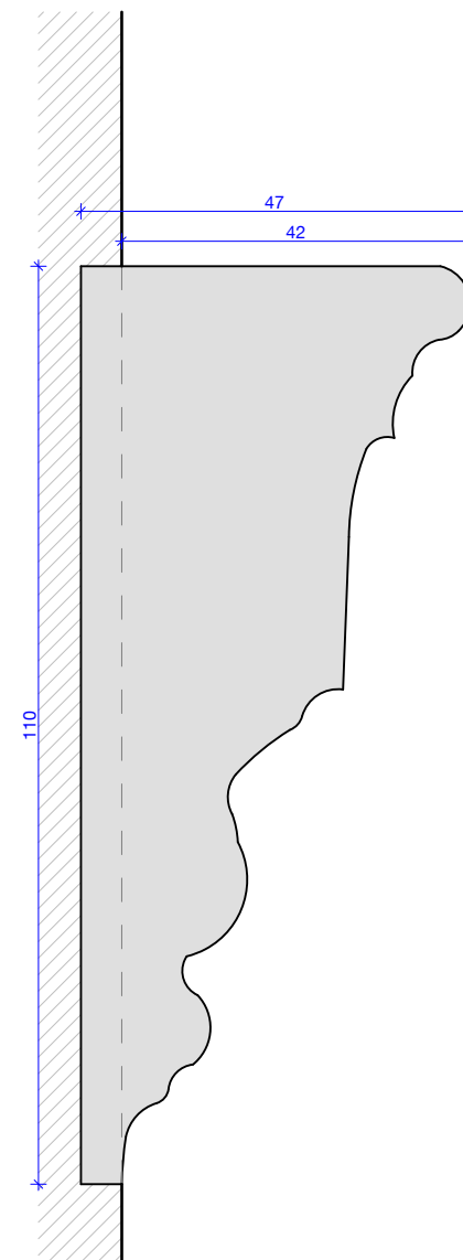
1:1 Dado Profile
