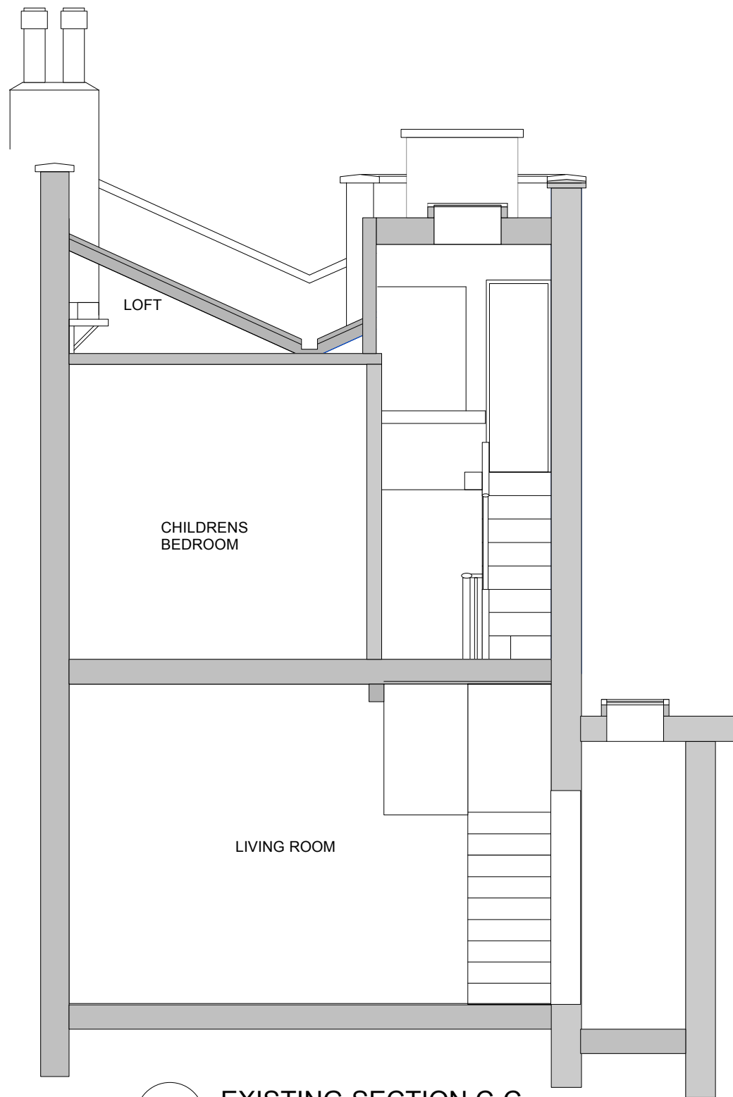
01 EXISTING SECTION C-C Scale: 1:50
