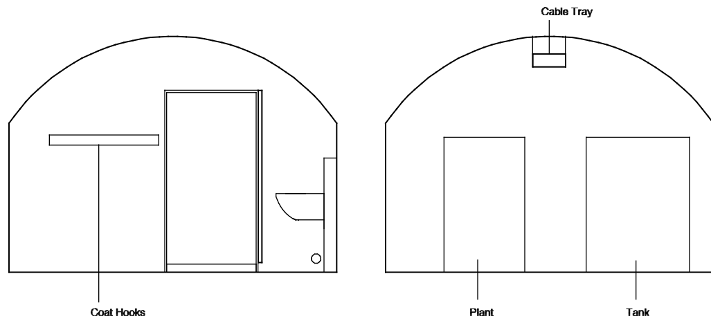
Elevation B
