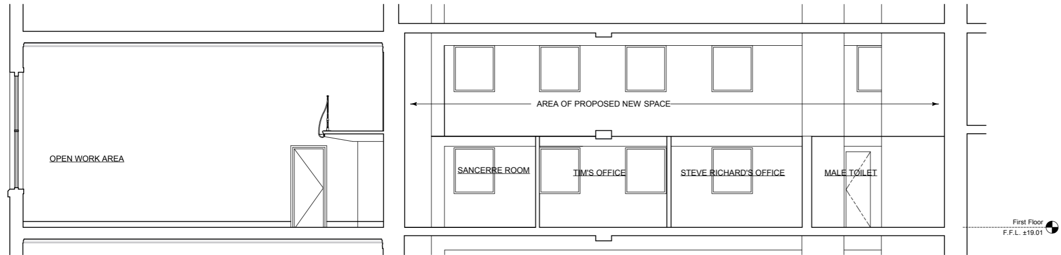
SECTION A-A
