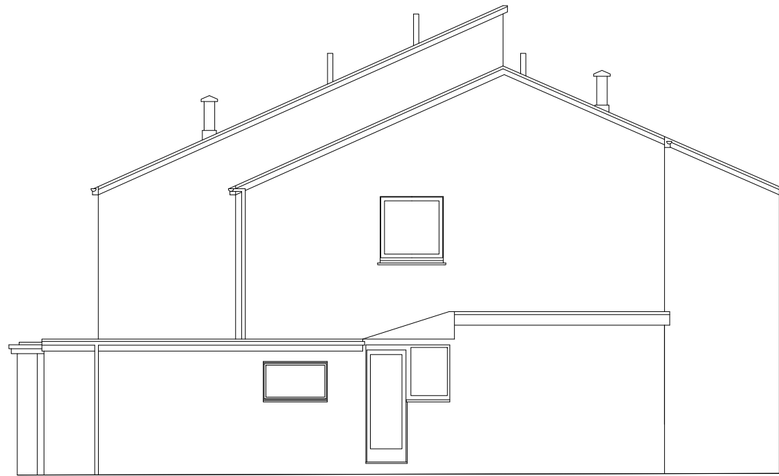
Elevation D - D
