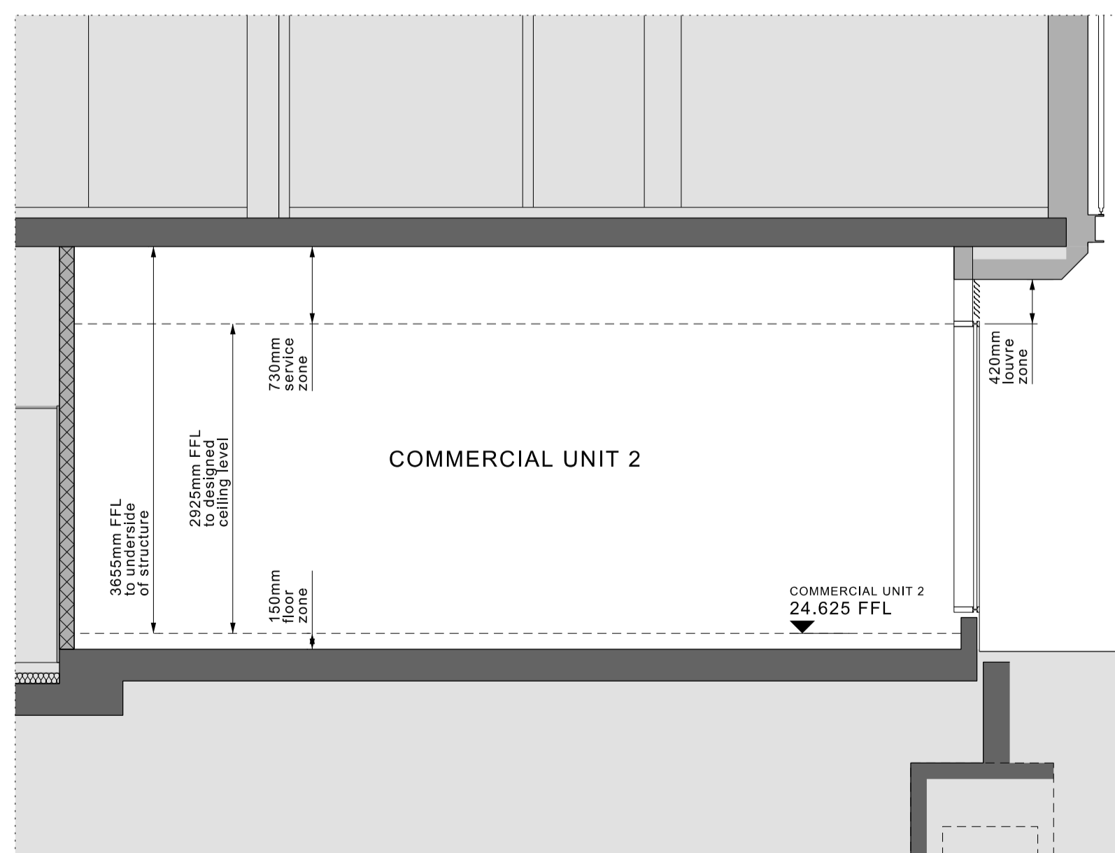
SECTION A-A
