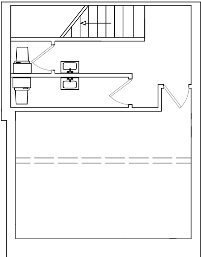
Existing Basement Scale: 1:100
