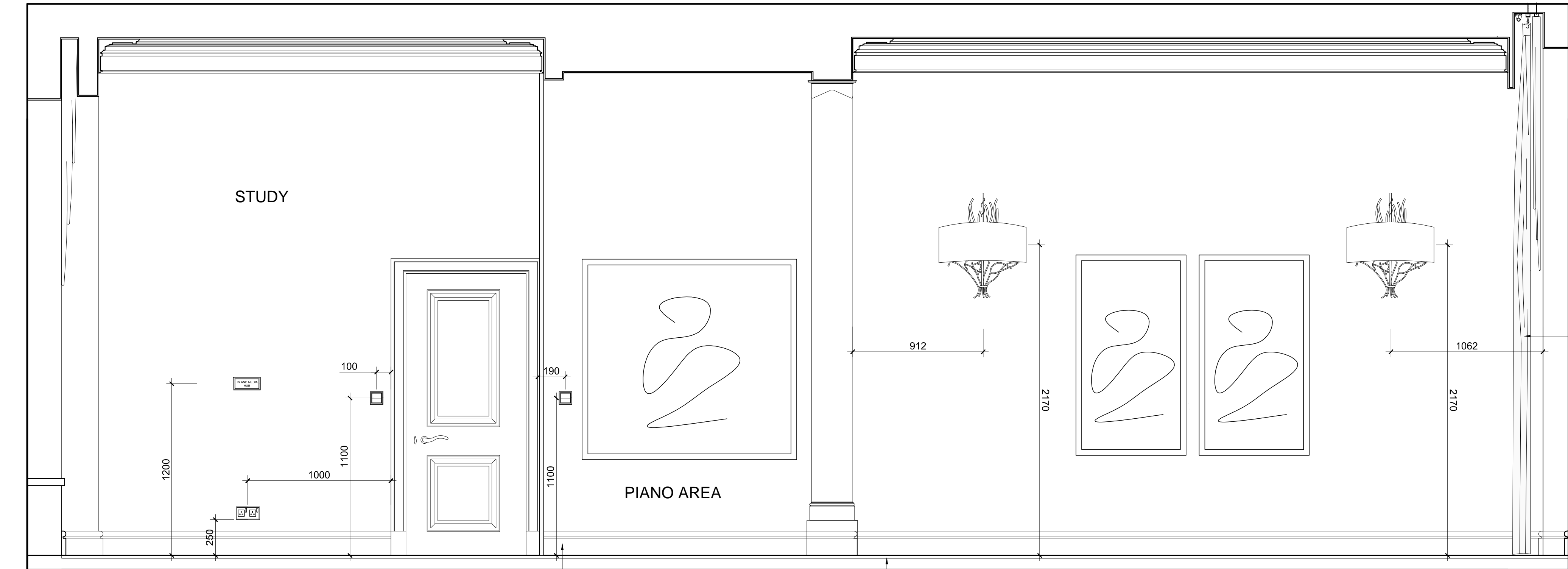
ELEVATION G
