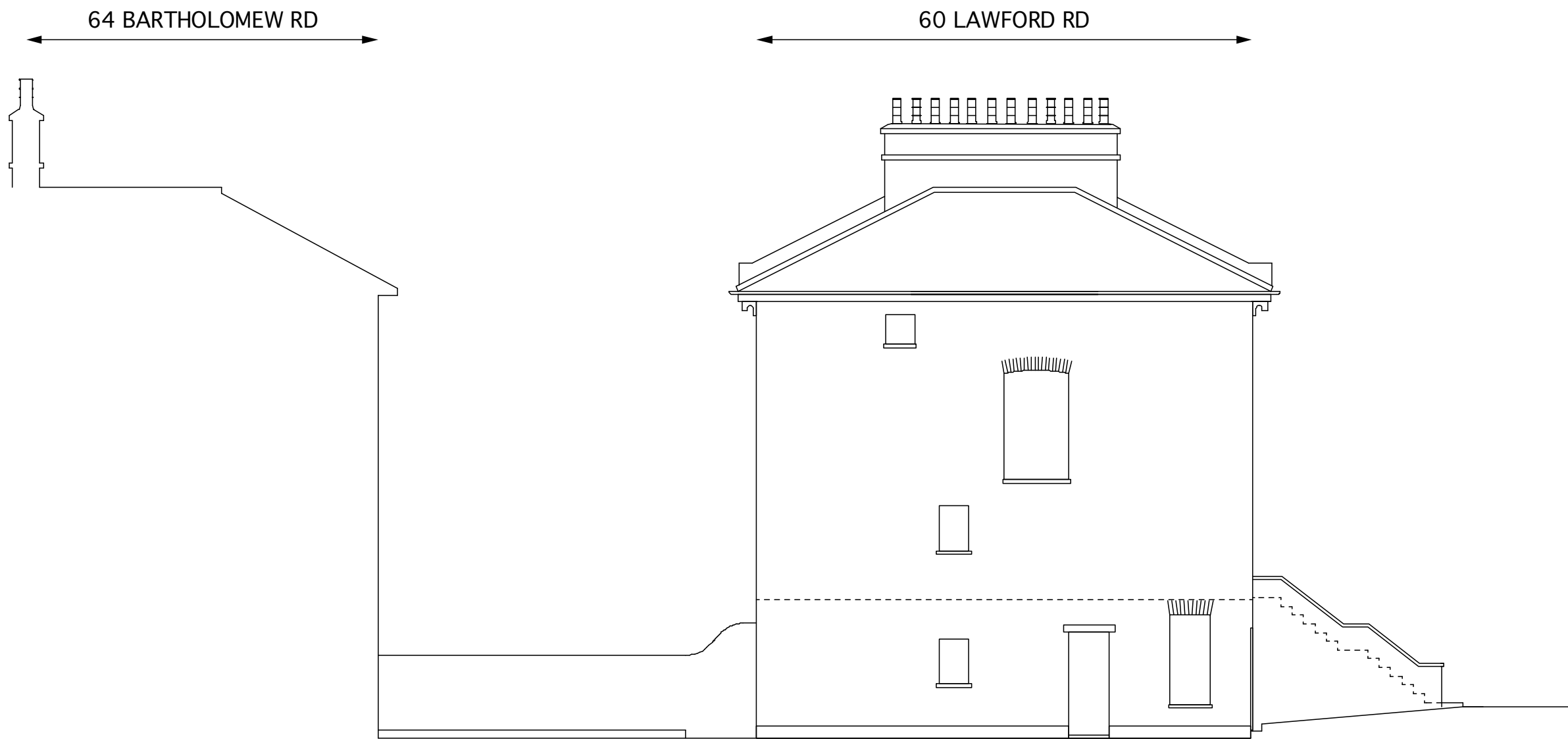
1 flank elevation Scale: 1:100
