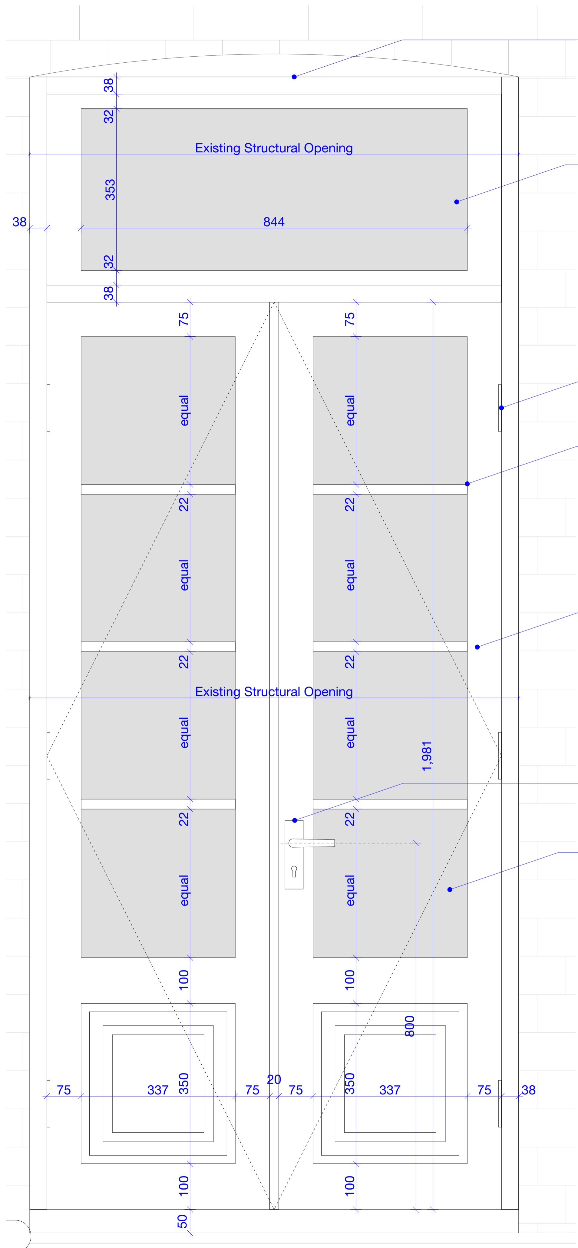
Elevation
