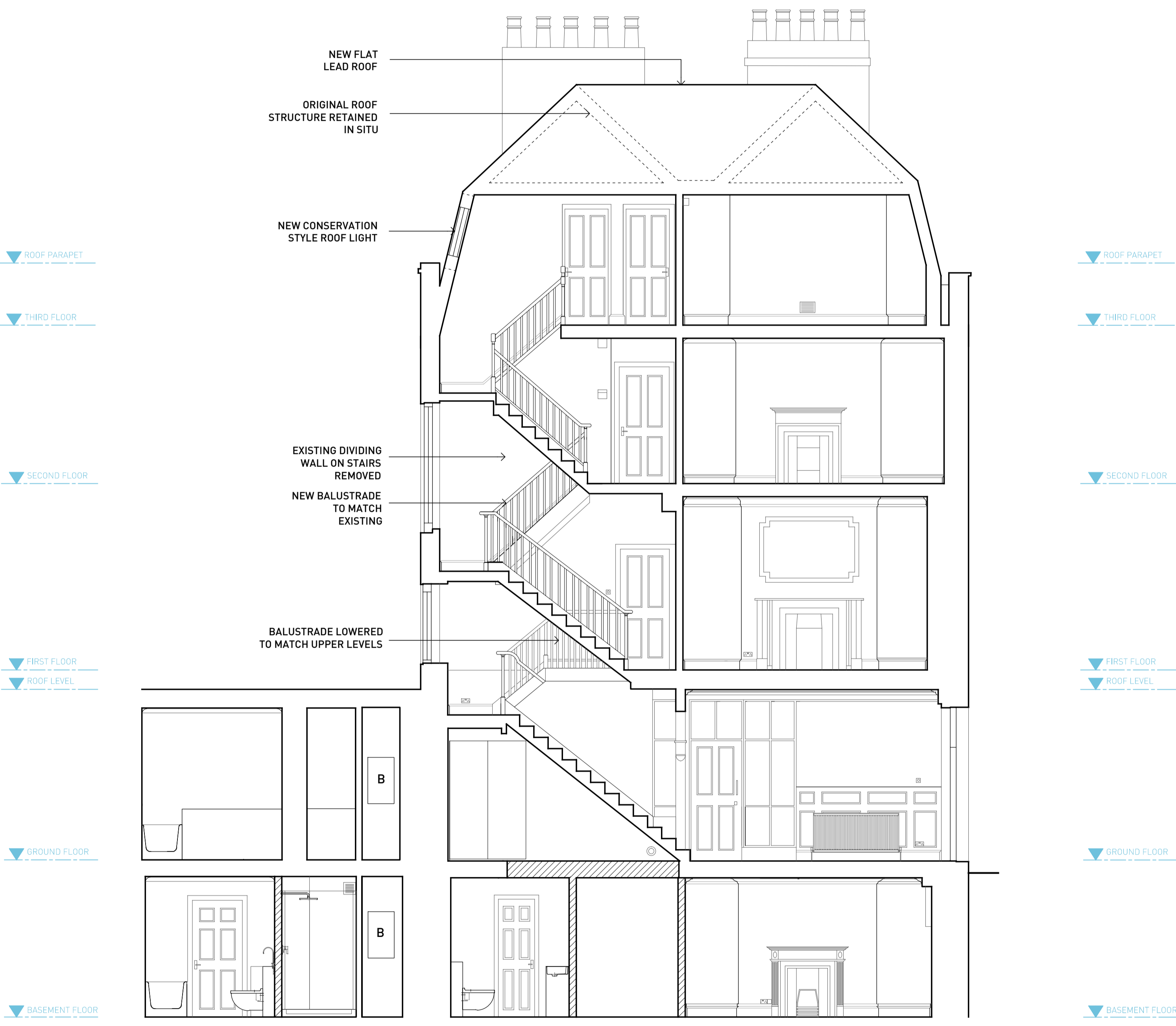
SECTION A-A
