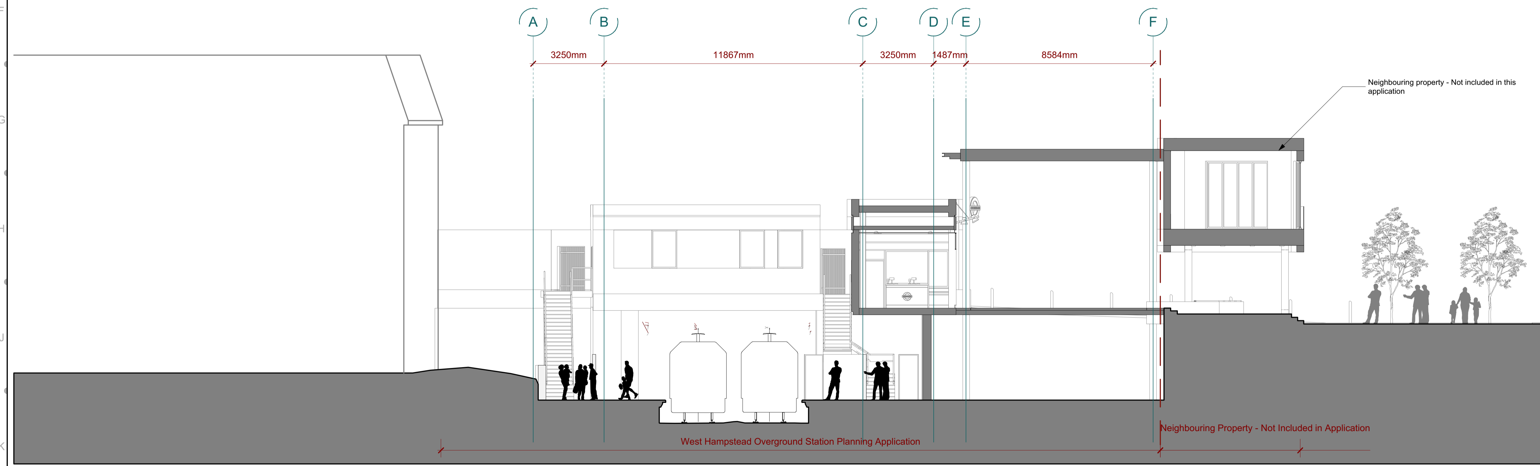
2 Section D-D Scale: 1:100
