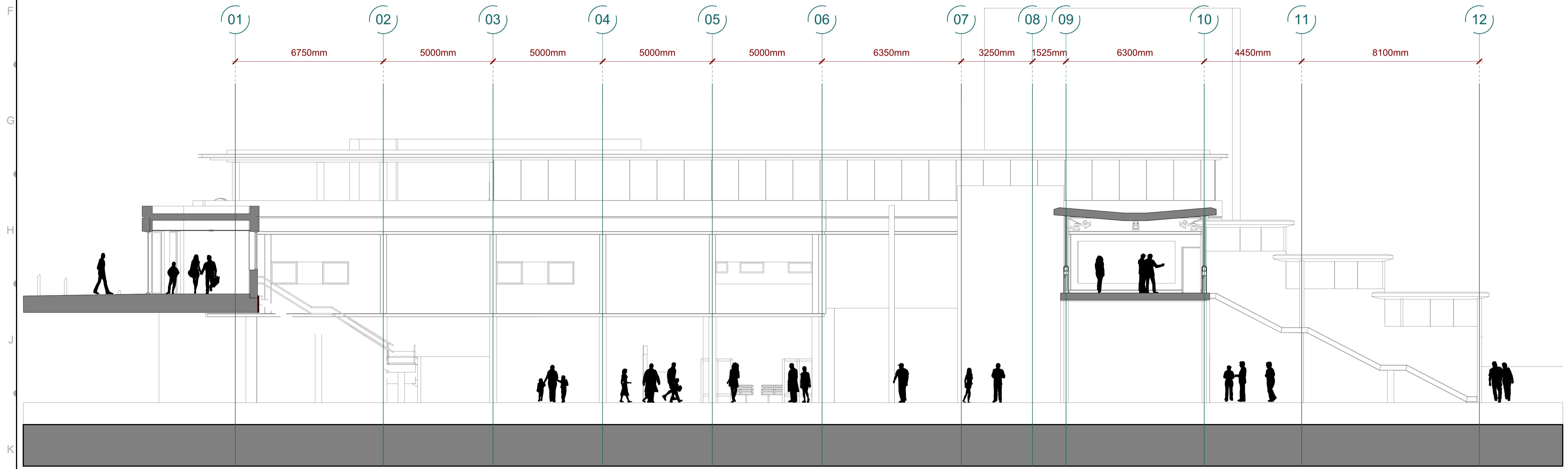
2 Section B-B Scale: 1:100
