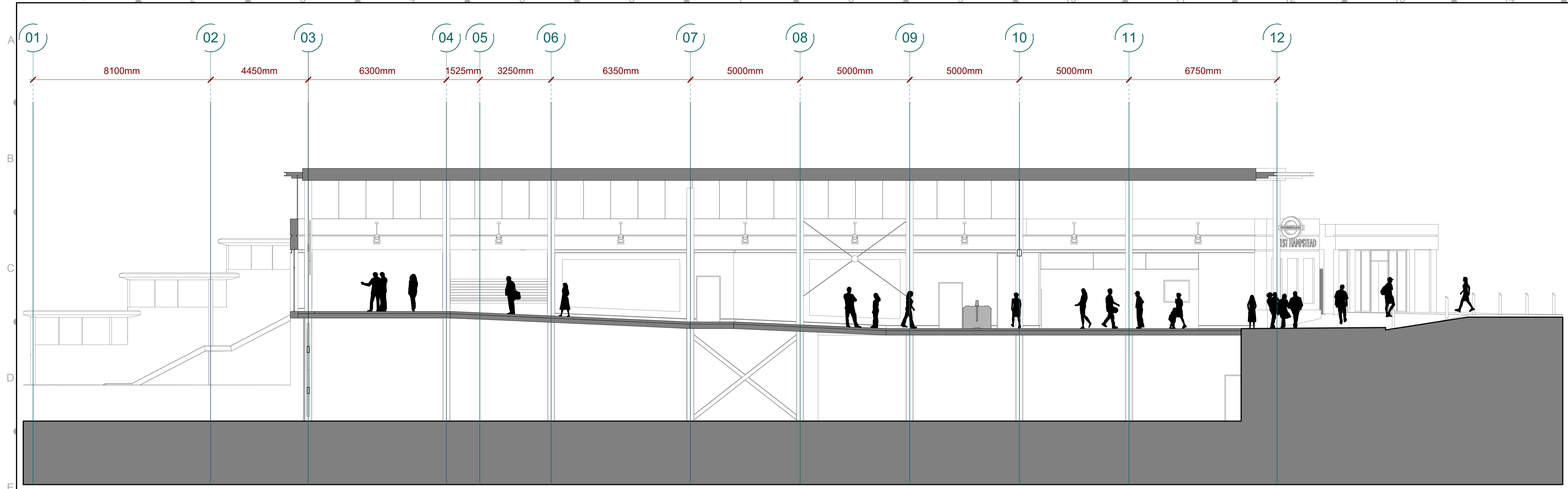
1 Section A-A Scale: 1:100
