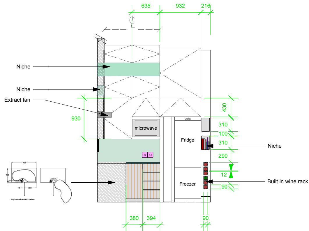
Elevation C 1:50 @ A3
