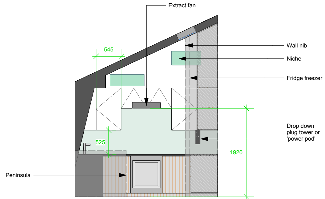
Elevation B 1:50 @ A3
