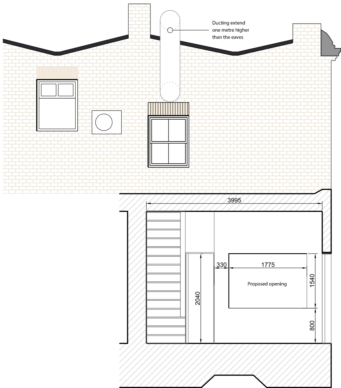
SECTION D-D
