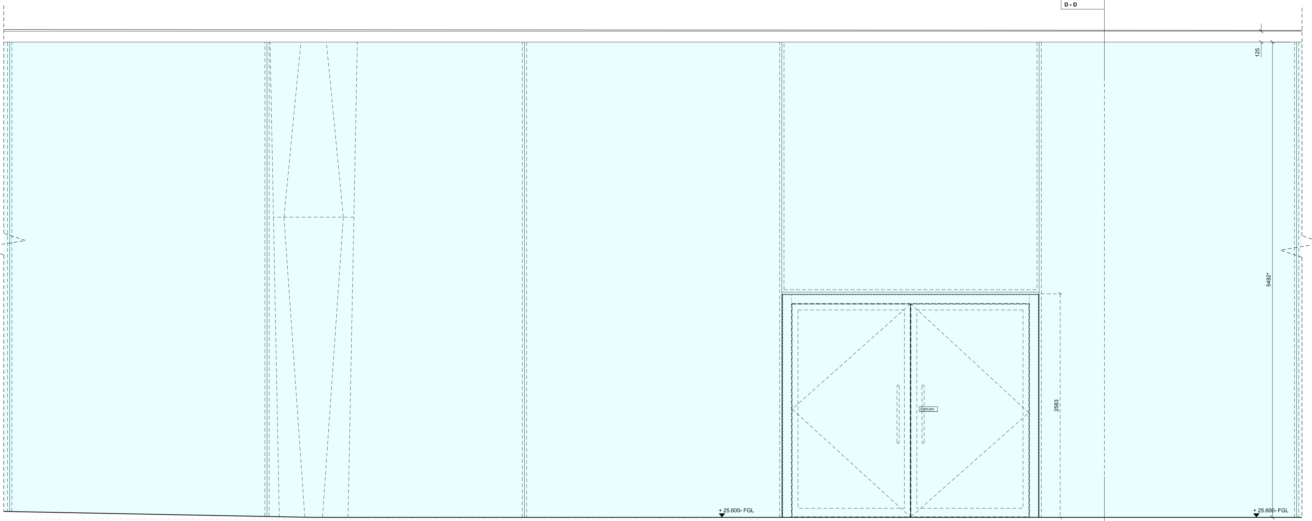
W0.004- N. Elevation 01 01 552-15452
