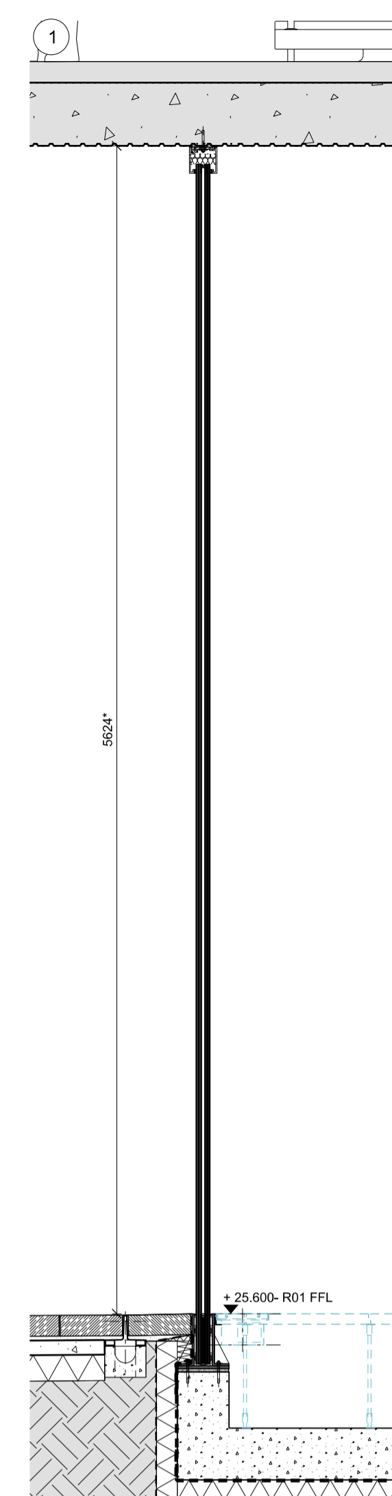
W0.004- Section DD 02 552-15452
