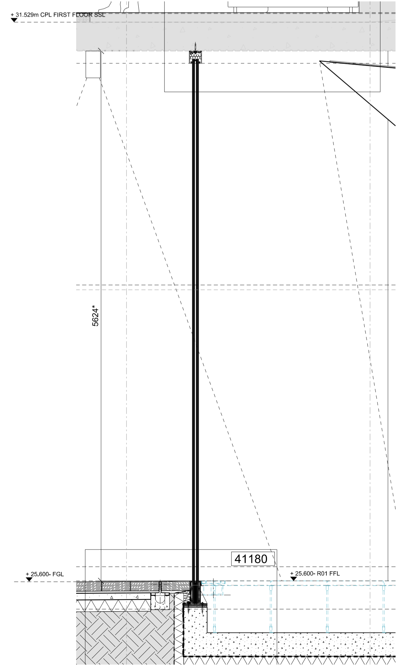
W0.004- Section DD
