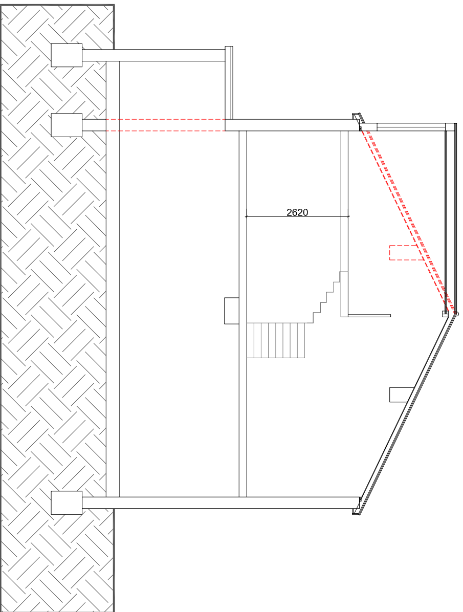
SECTION A-A
