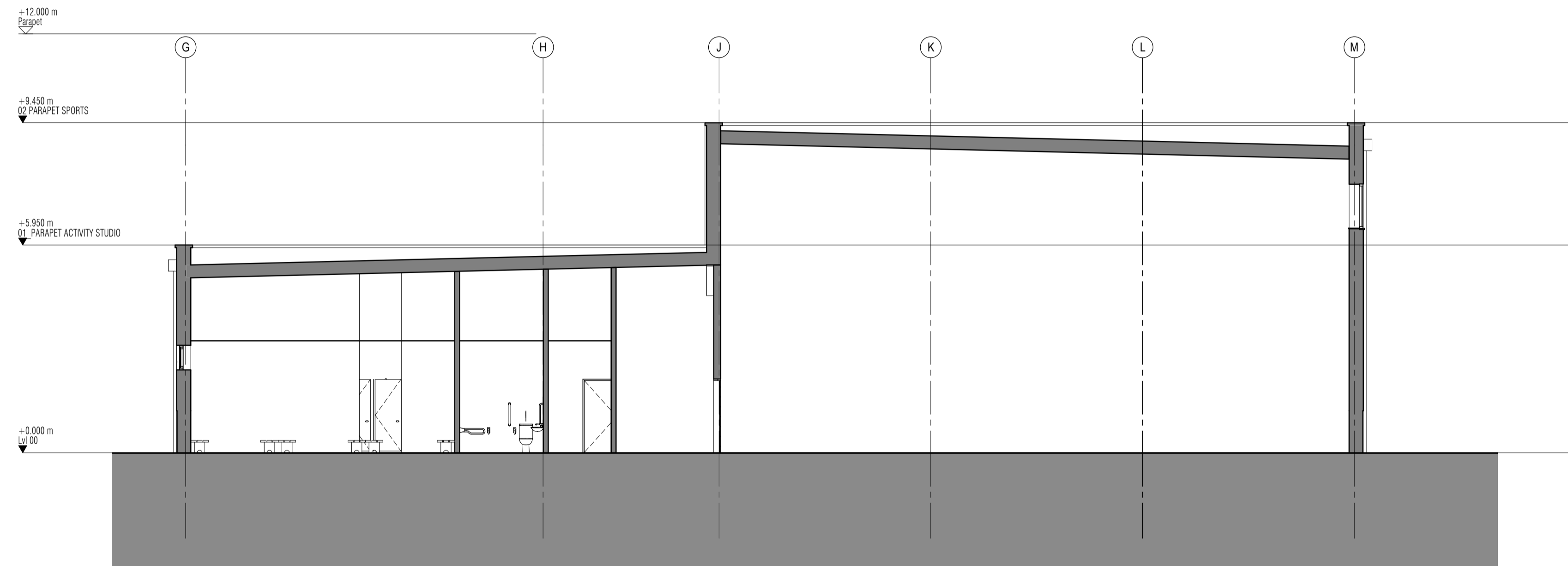
1 SECTION DD JW-310 / 1:100
