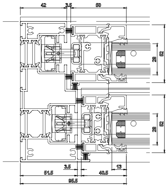
4 jamb detail
