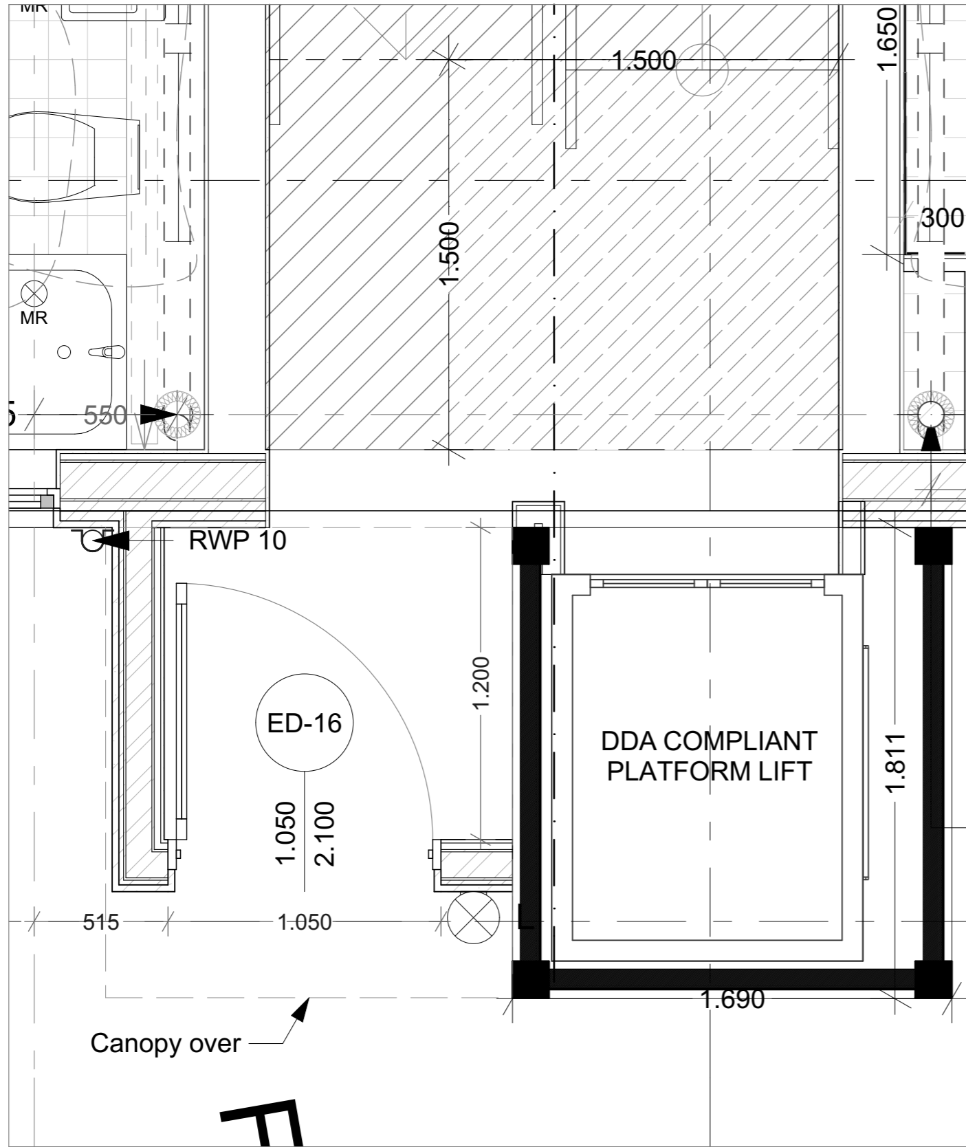
3. PLAN 1:20
