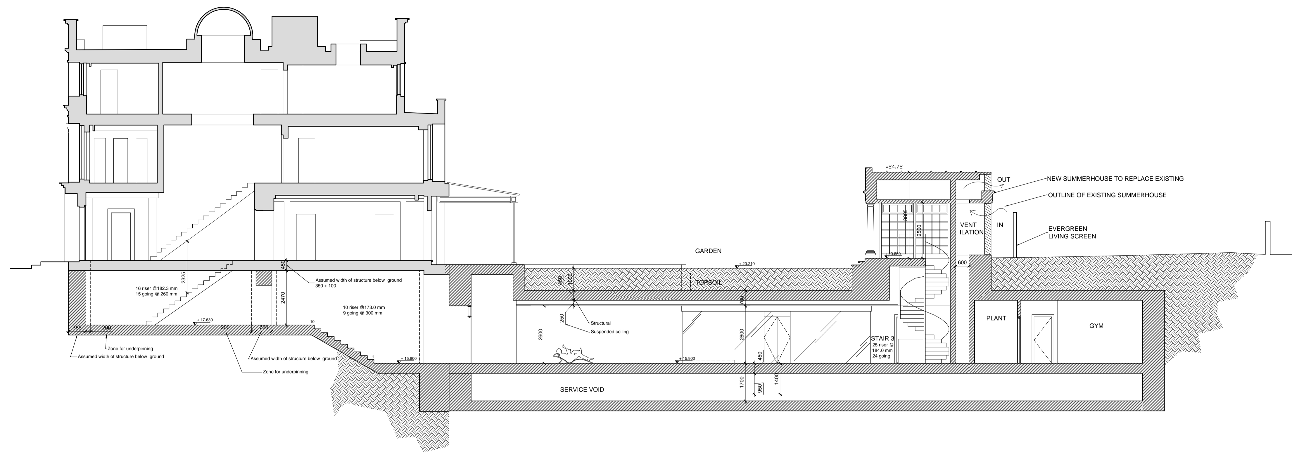
SECTION A-A
