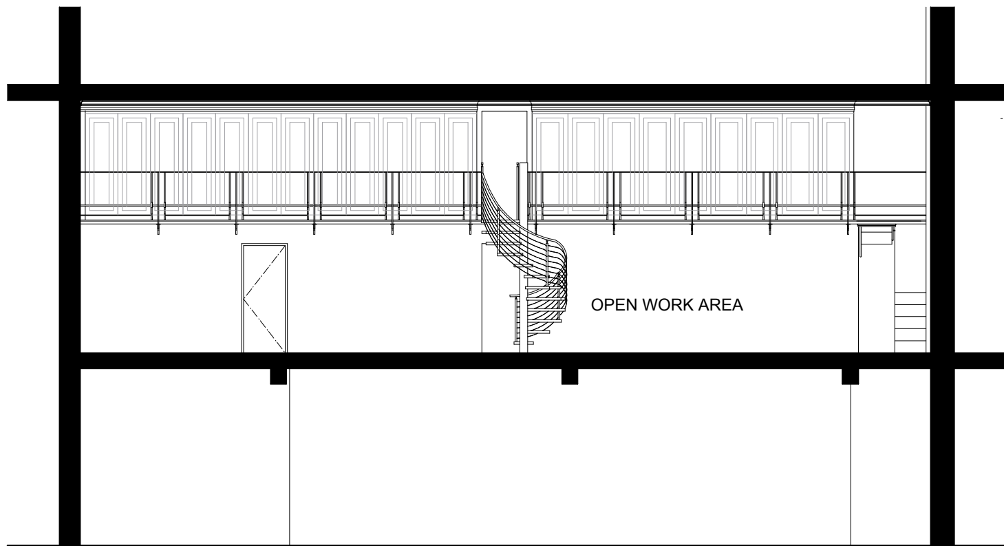
SECTION A-A
