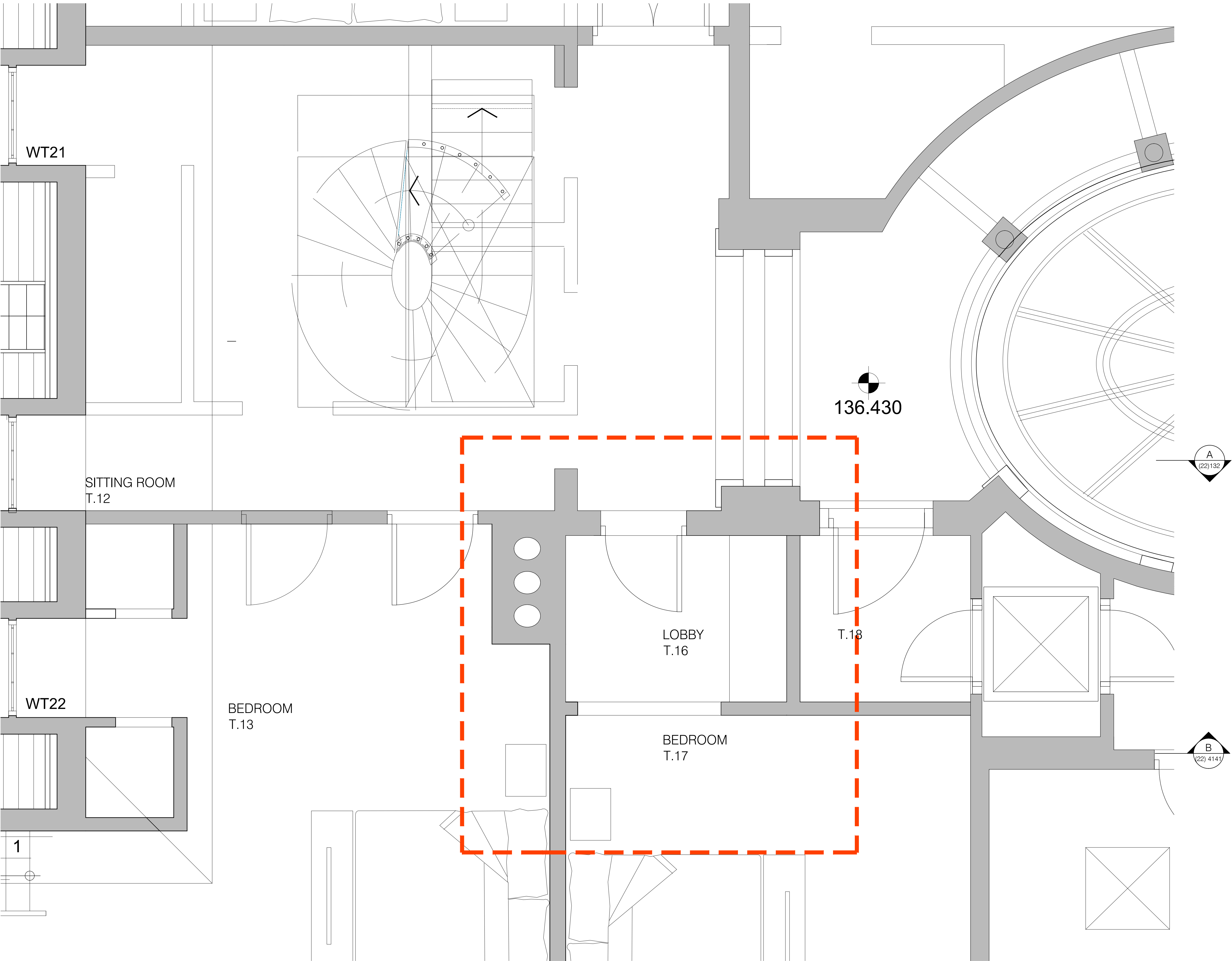
T13 LANDING/TEA BAR PLAN Scale: 1:20 @ A1
