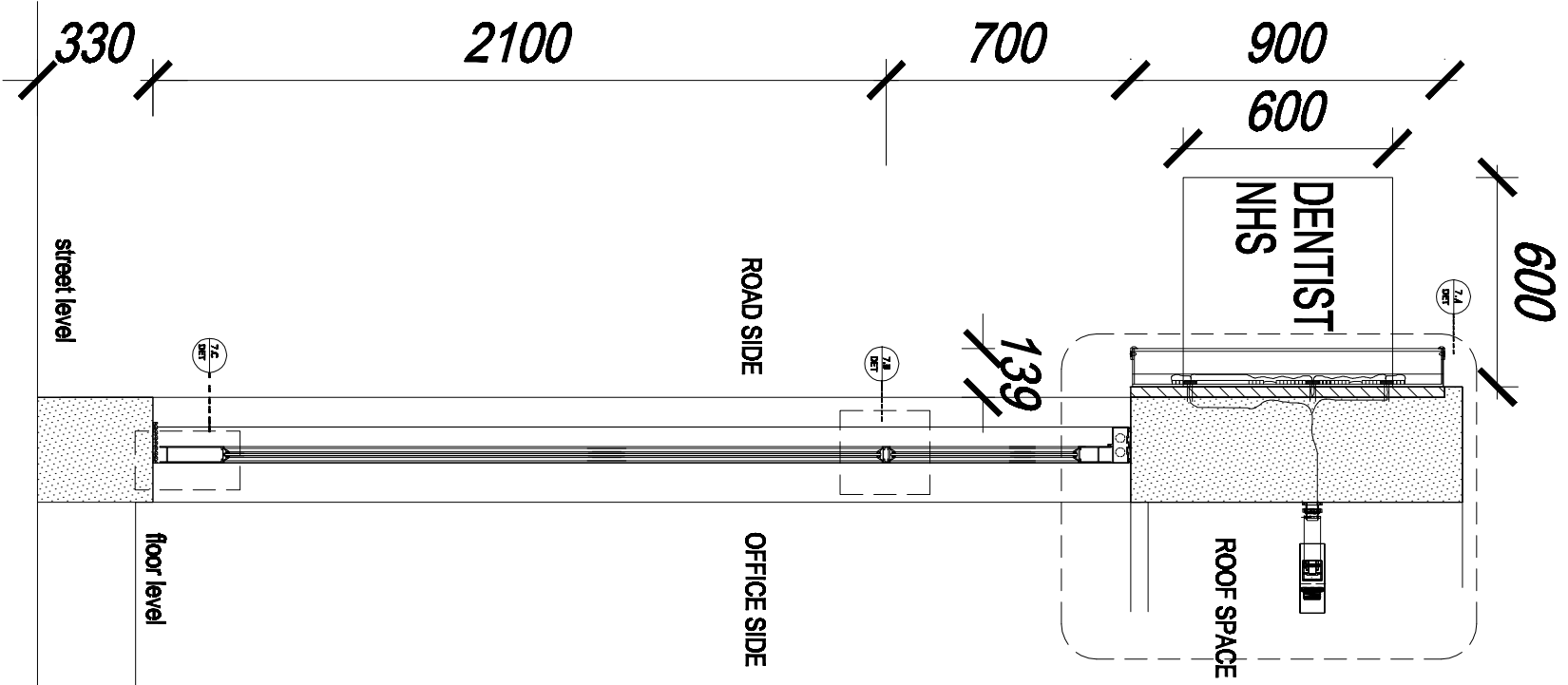
SECTION A-A 1:20
