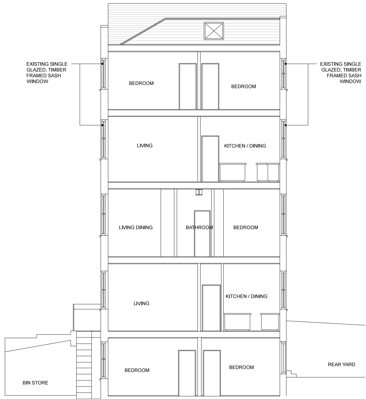
SECTION A-A
