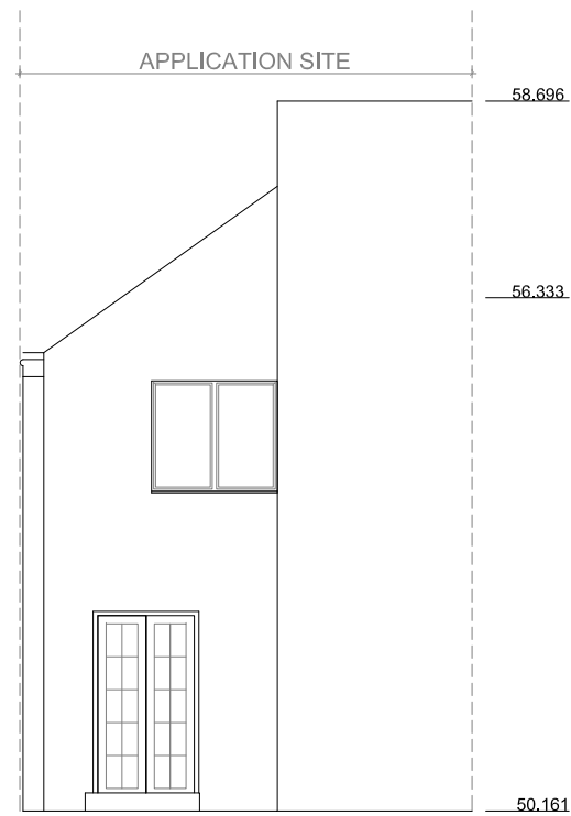
Elevation 5 Existing
