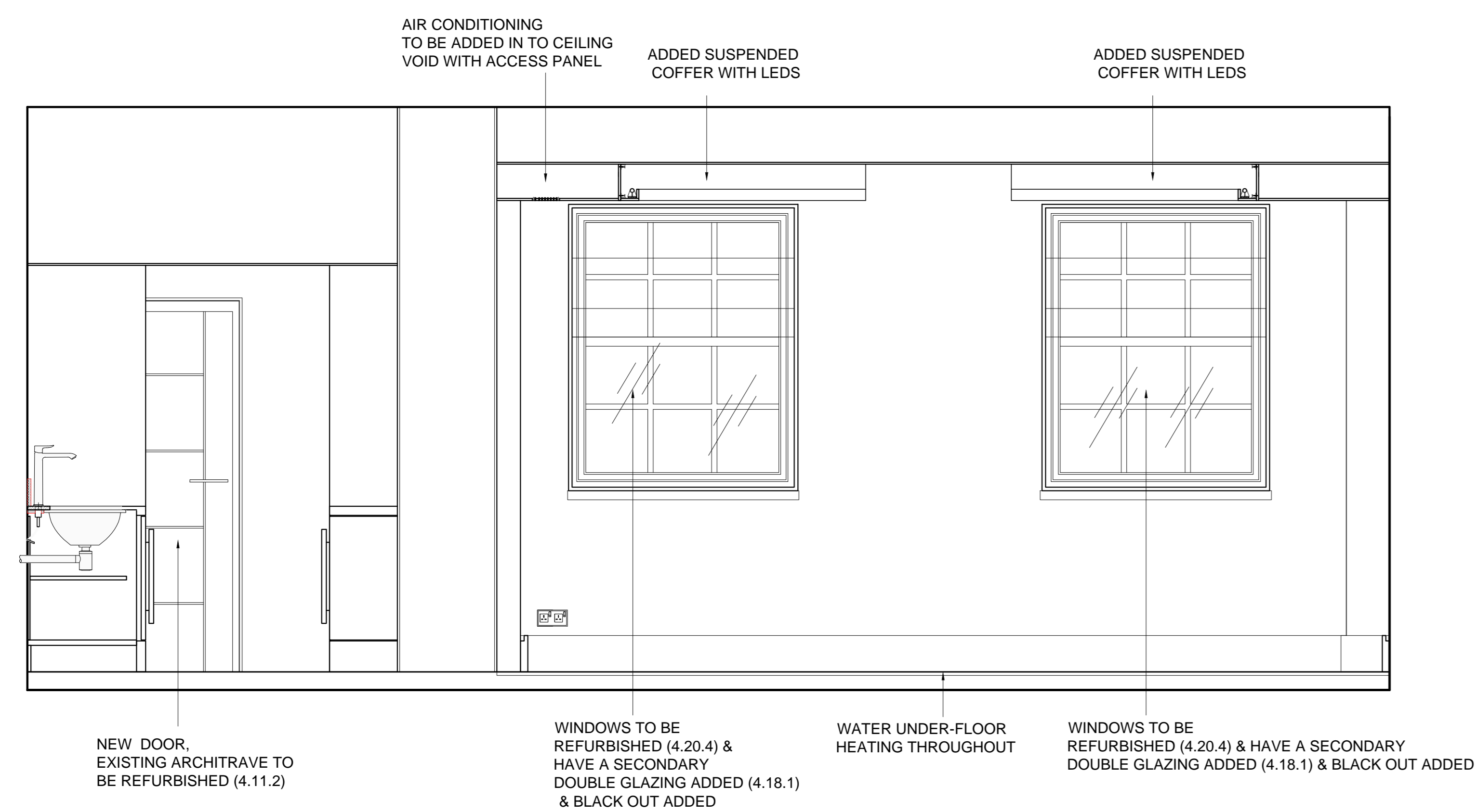
ELEVATION E
