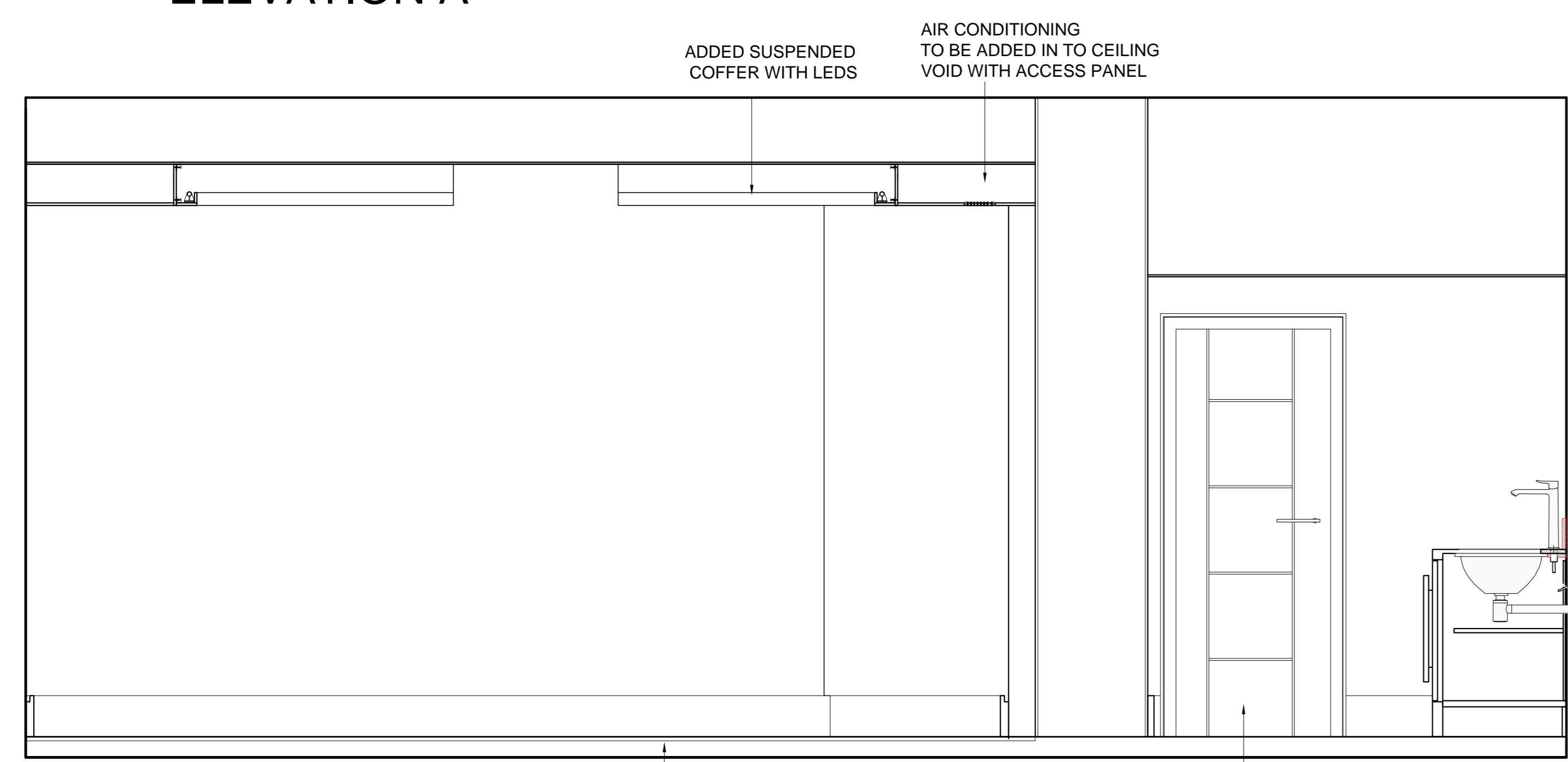
ELEVATION A
