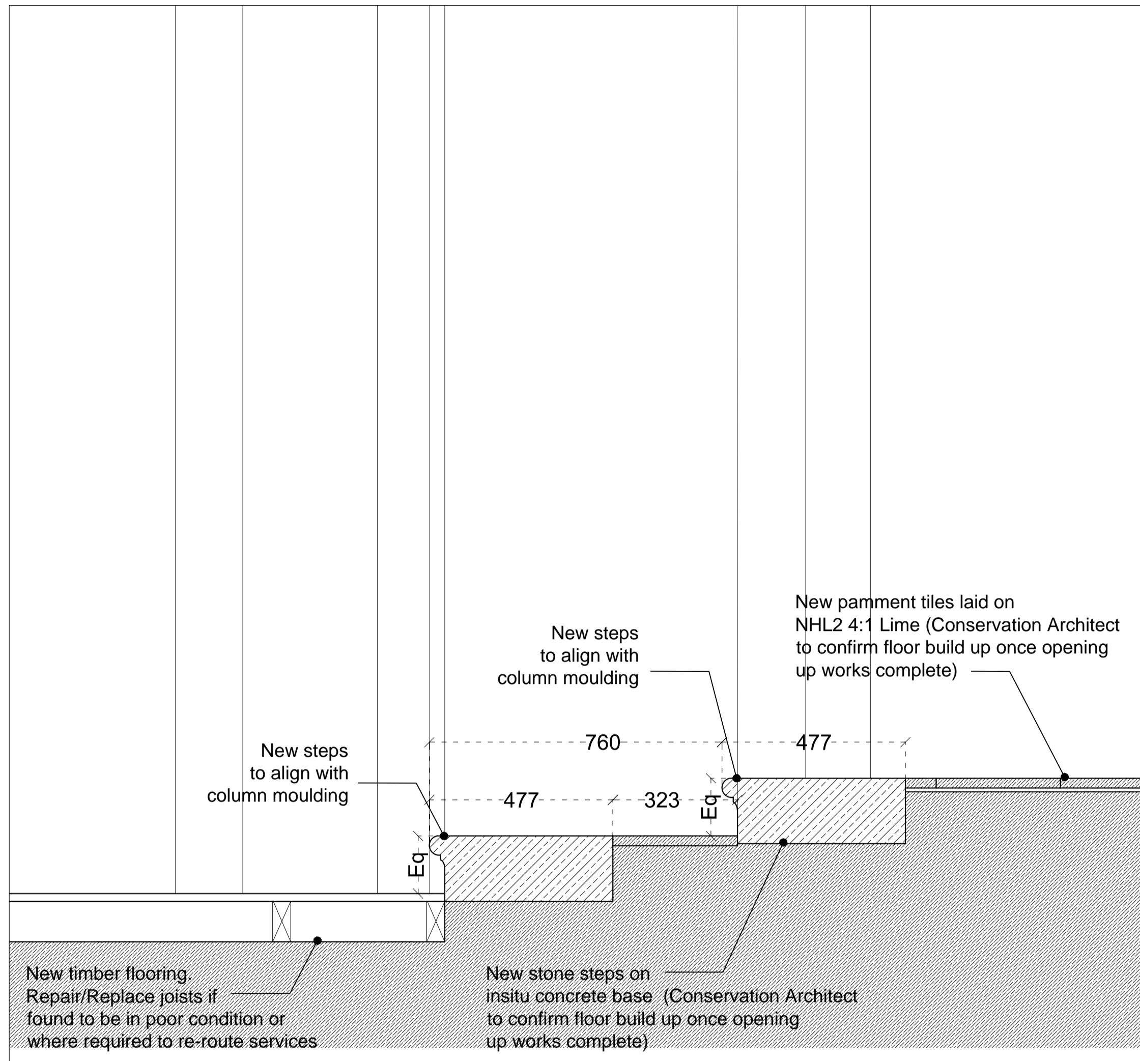
Section A-A 1:10@A1 / 1:20@A3
