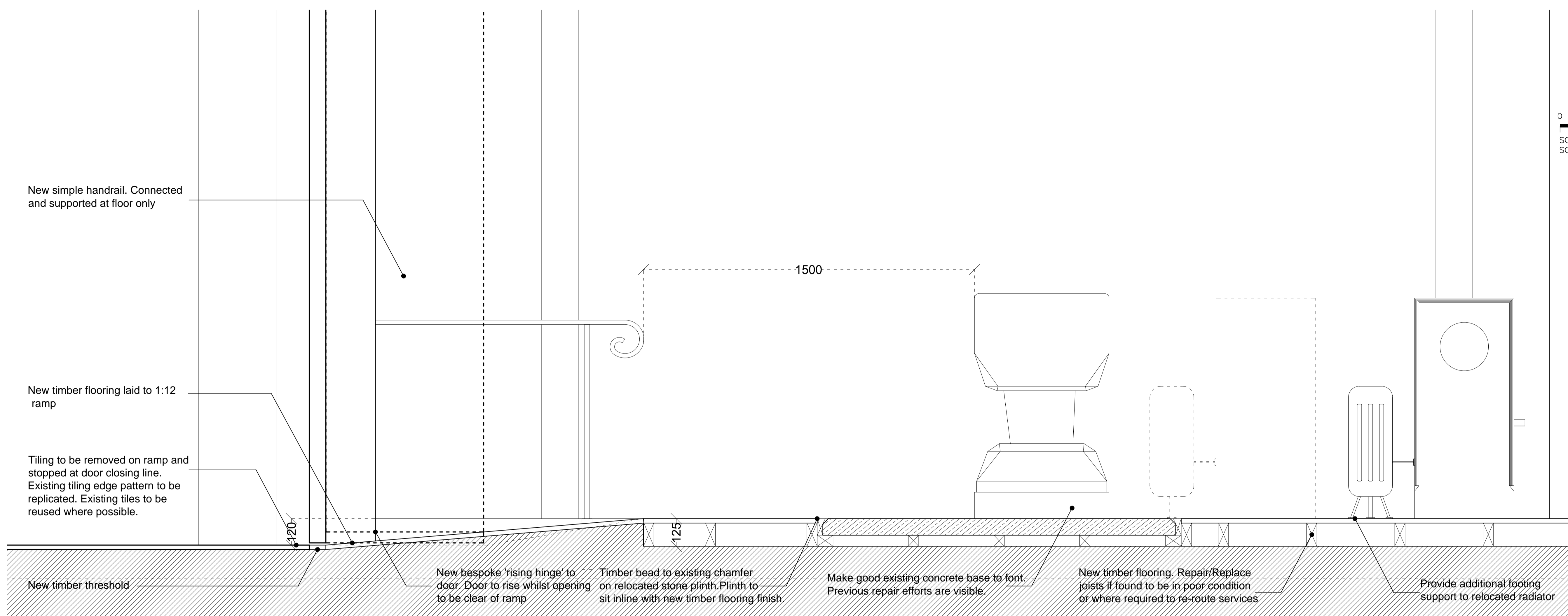
Section 1:10@A1 / 1:20@A3
