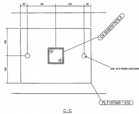
C - C
