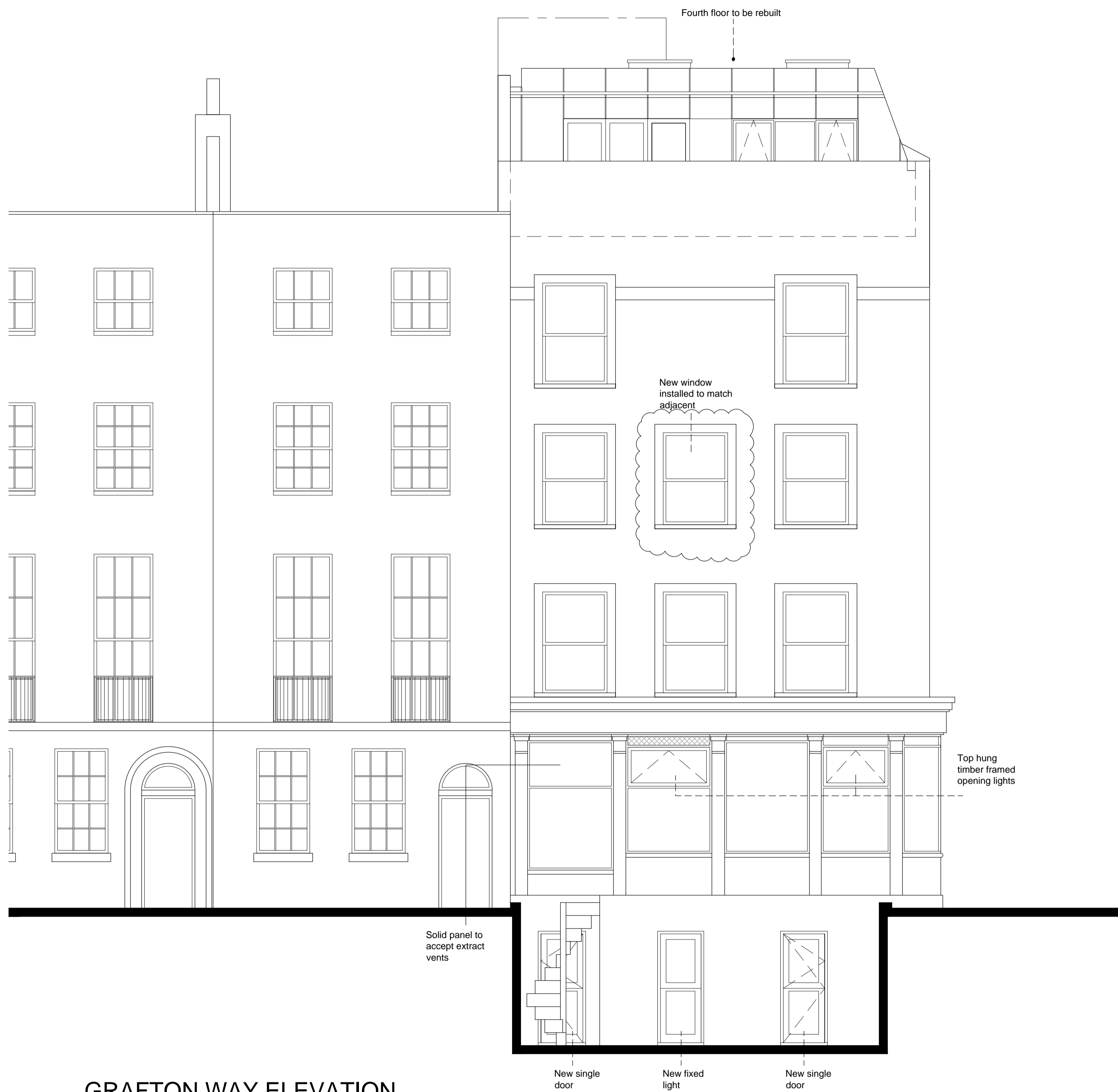
GRAFTON WAY ELEVATION
