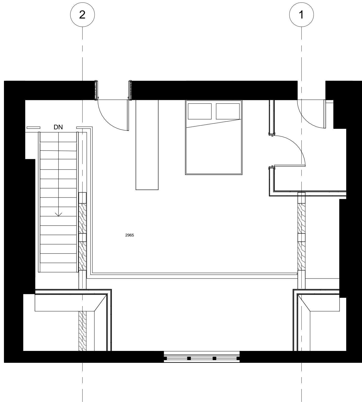
1 Fifth Floor(entrance)_Existing 1 : 50
