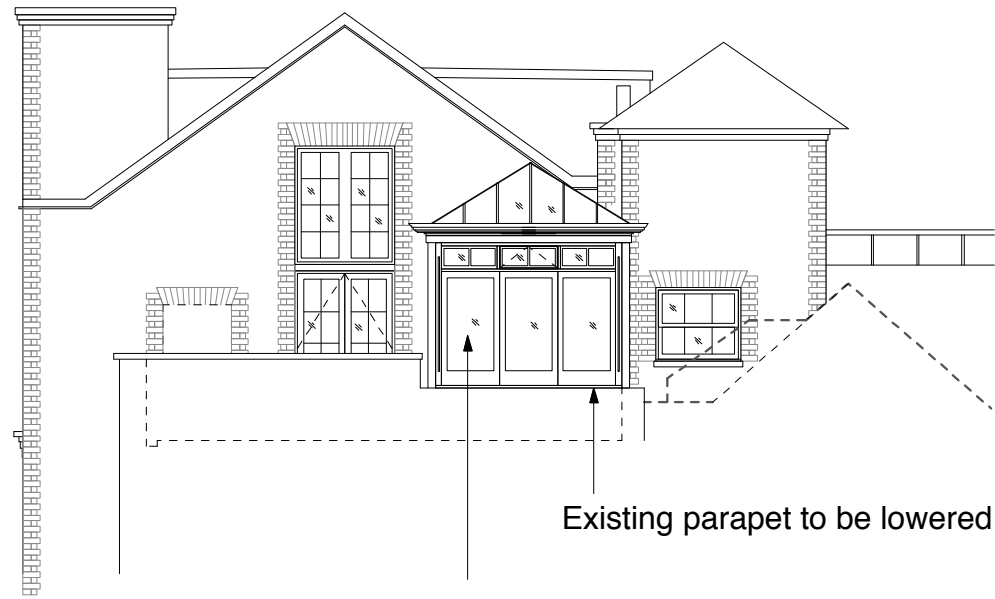
Elevation B
