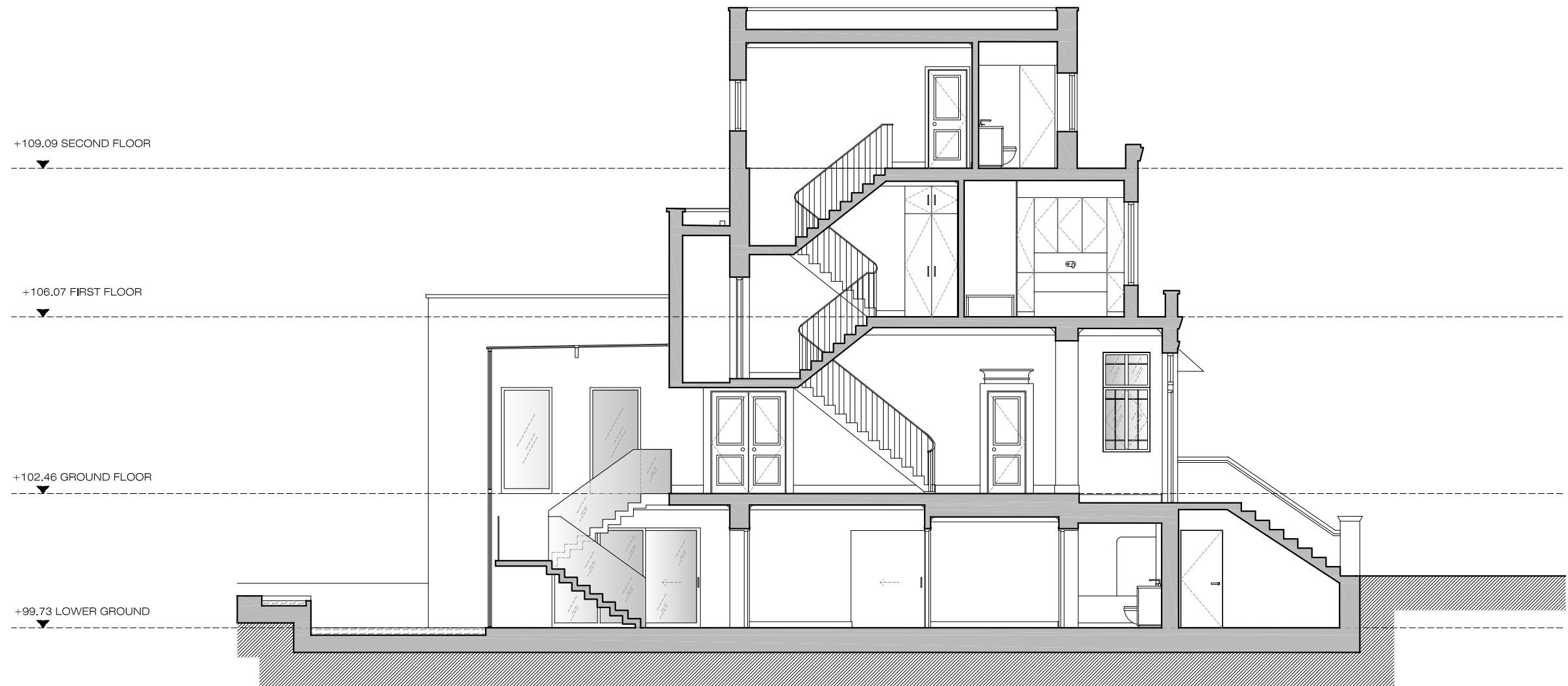
01 Section AA scale: 1:100 14_09
