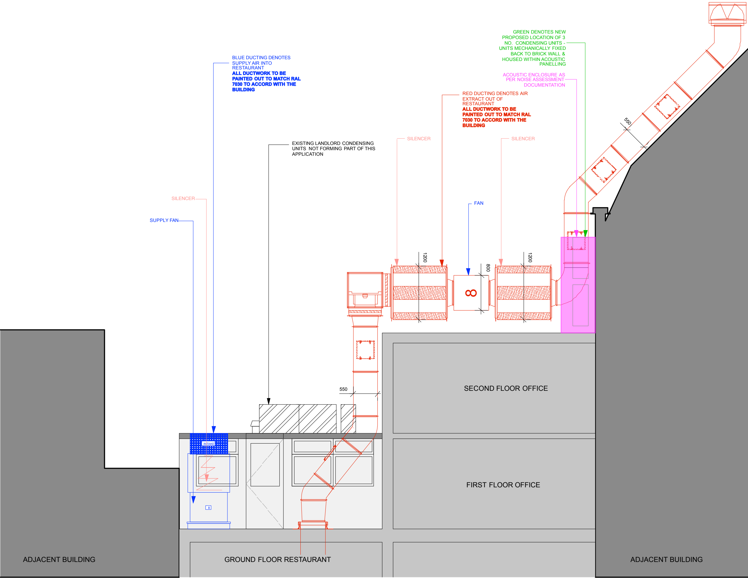
789 - ELEVATION AA SCALE 1:50 @ A3
