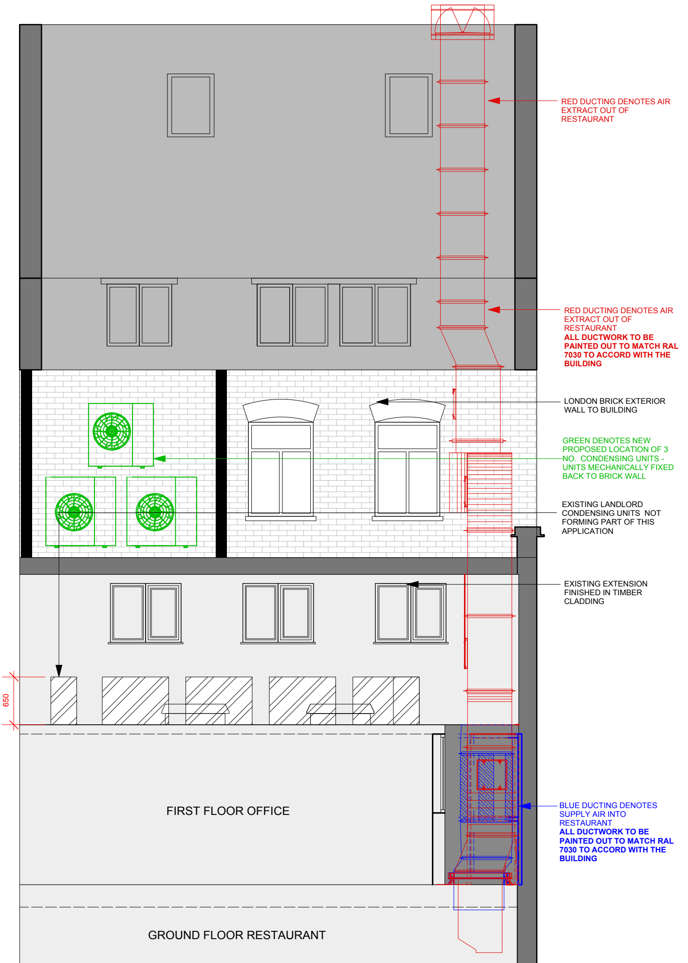
789 - ELEVATION BB SCALE 1:50 @ A3
