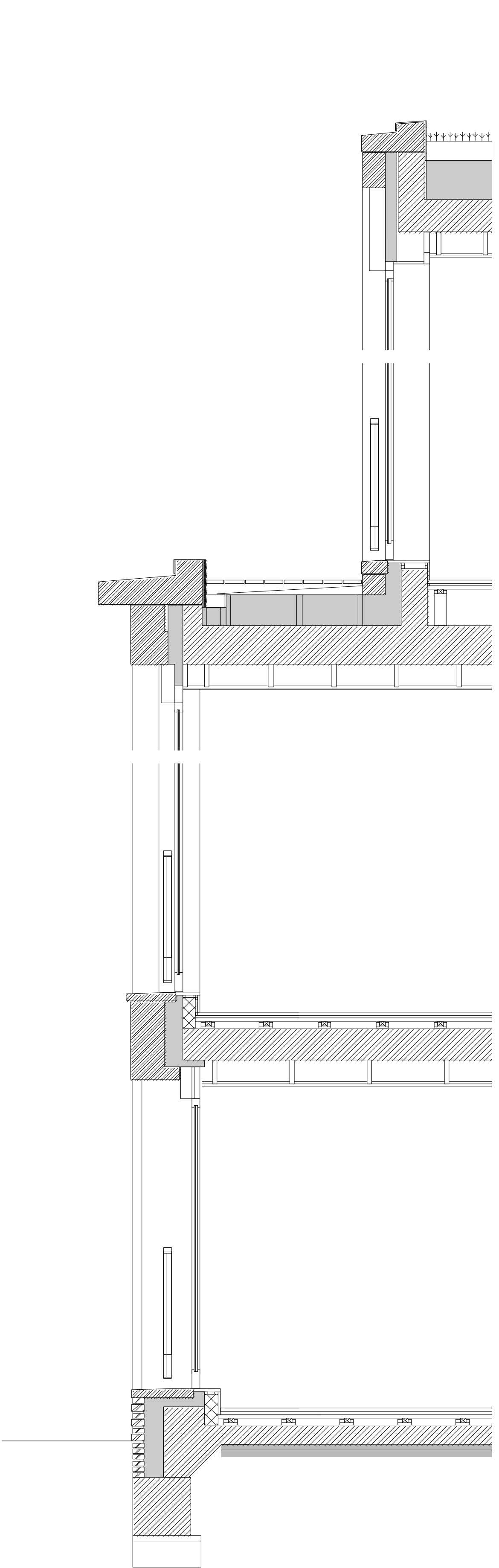
Section D 1:25
