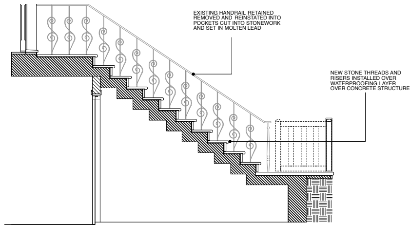
01 SECTION 340 1.20
