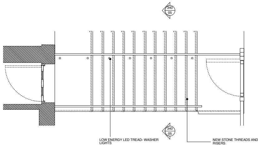
03 PLAN 340 1.20
