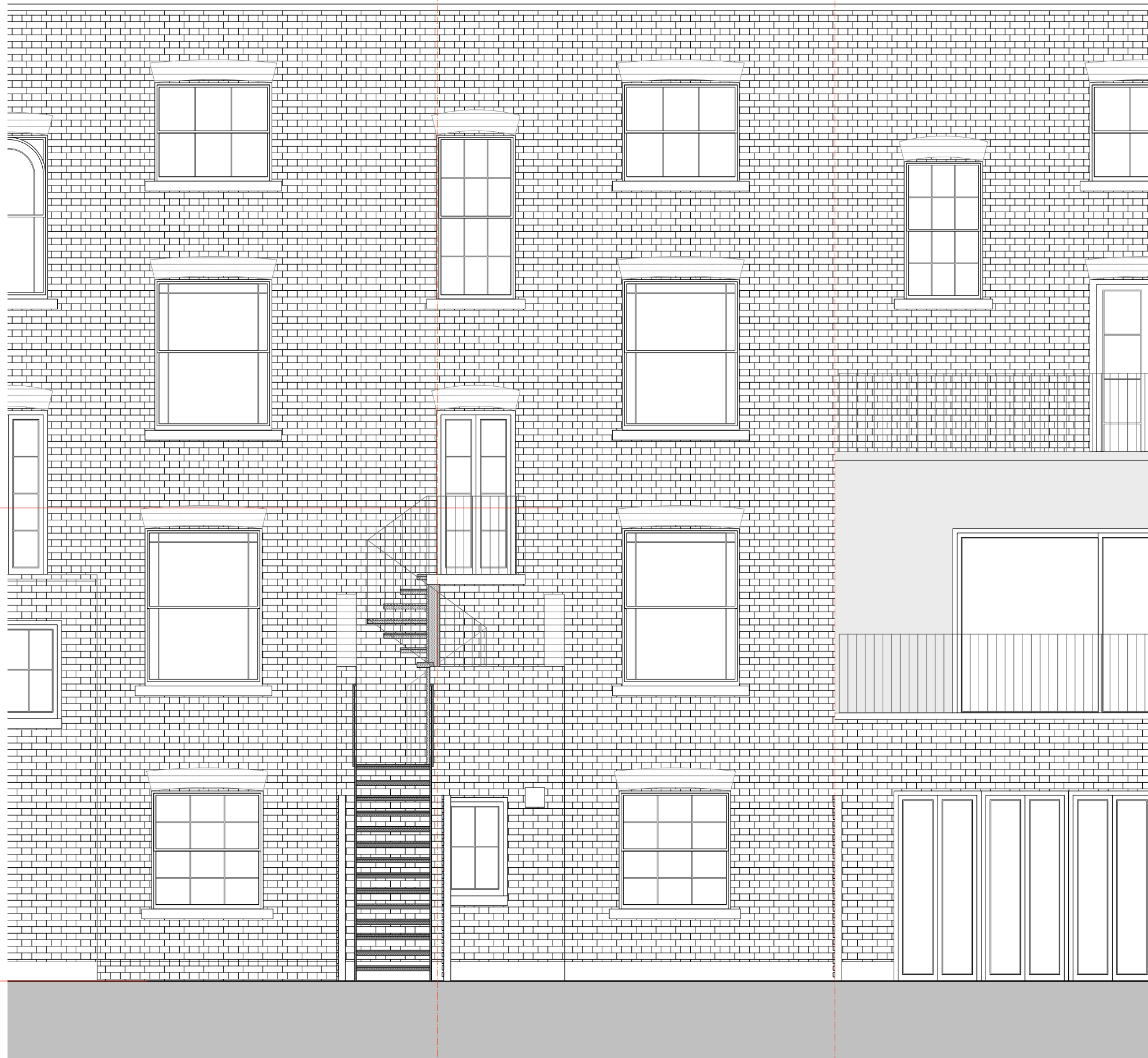
1 EXISTING REAR ELEVATION Scale: 1:25
