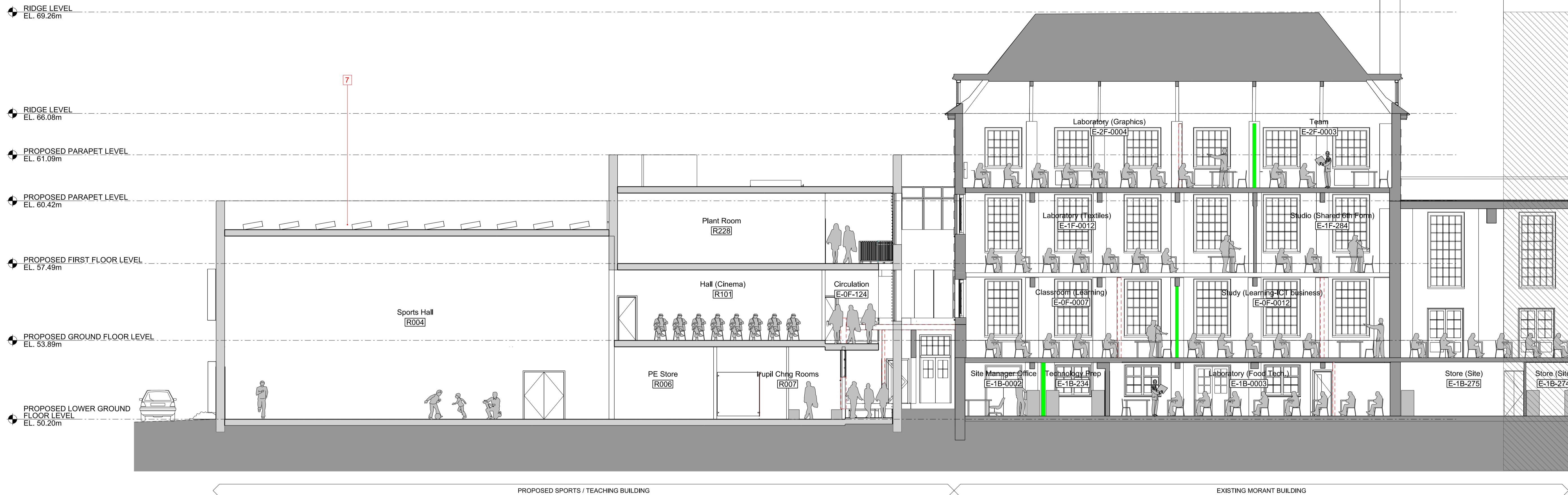
01 SECTION BB 1:100
