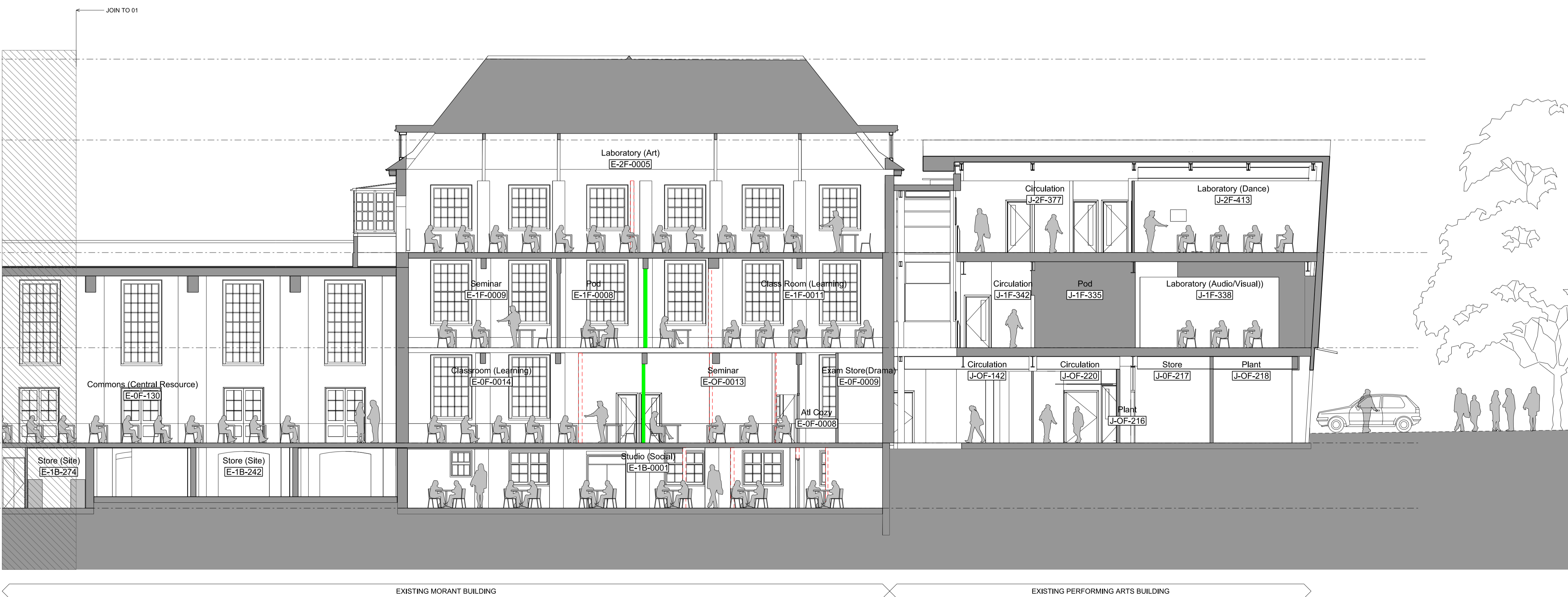
02 SECTION BB 1:100
