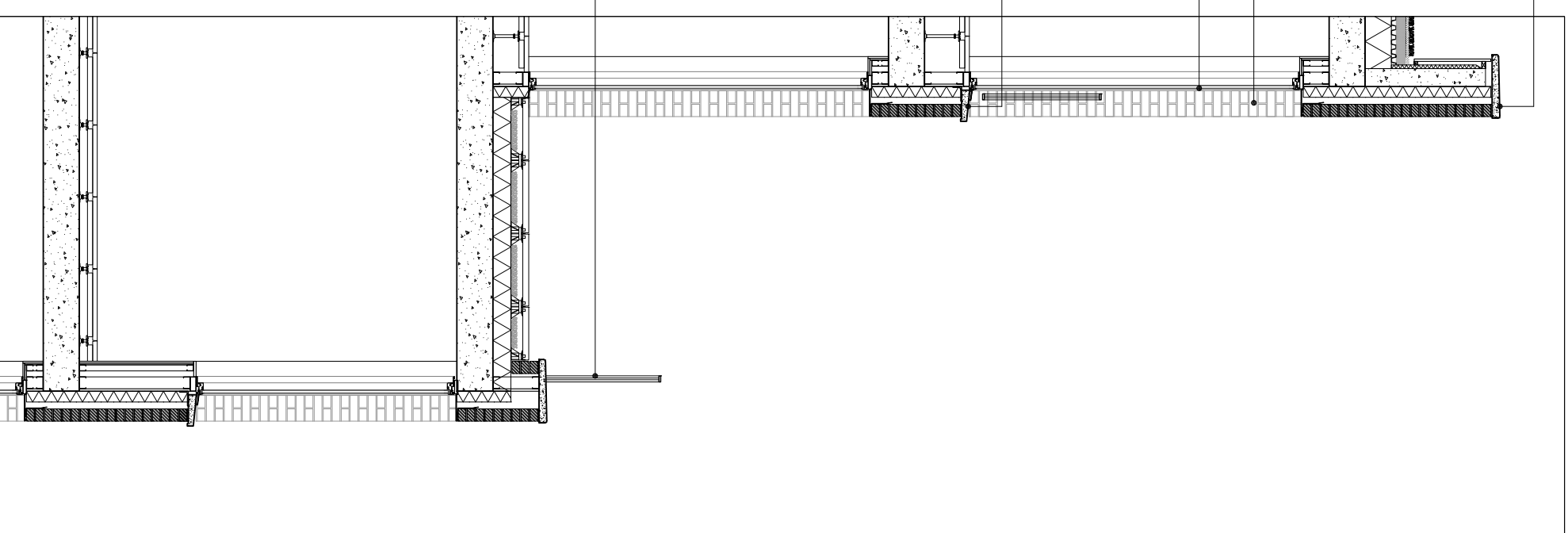
Section A-A
