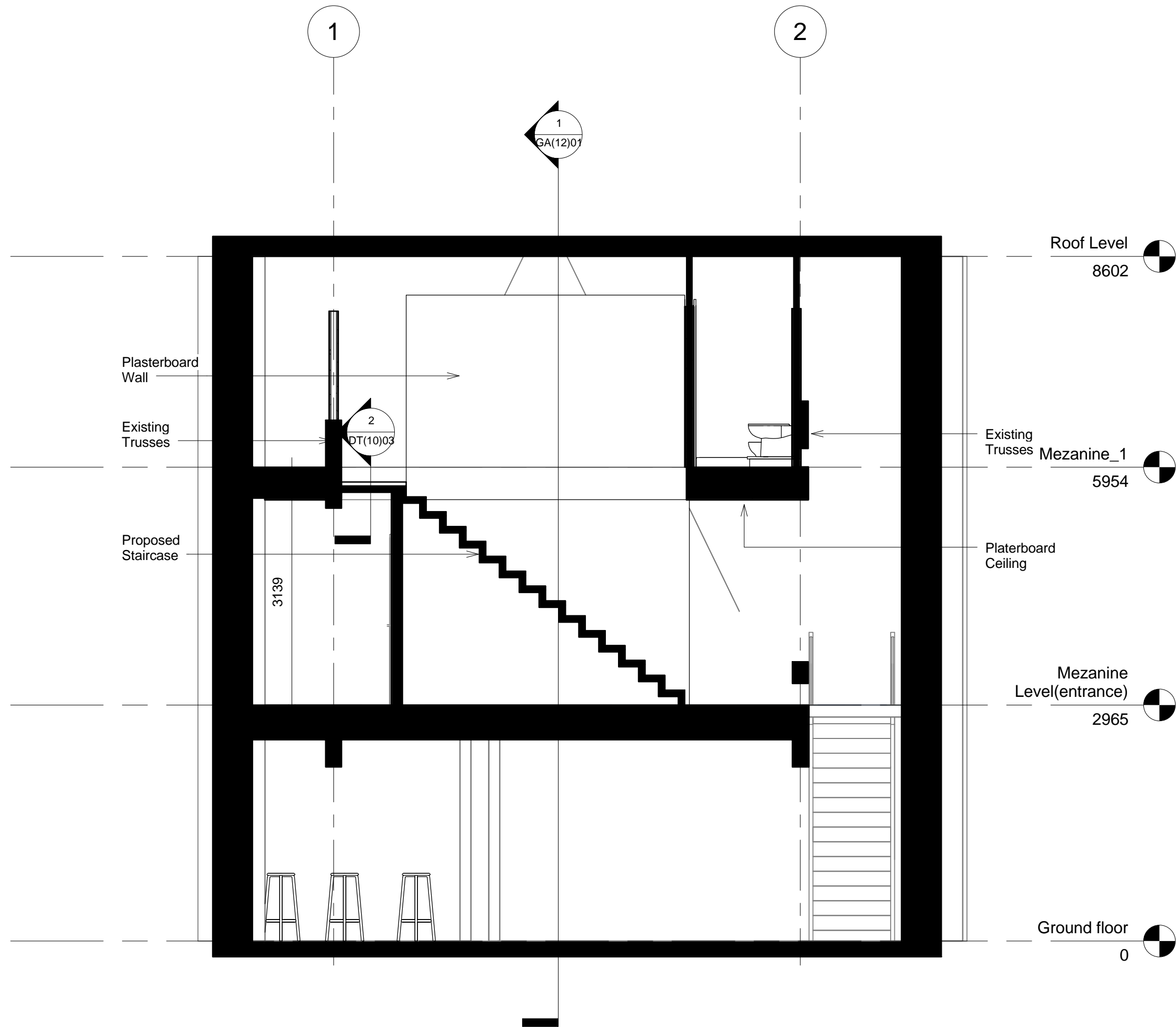
1 Section CC 1 : 50
